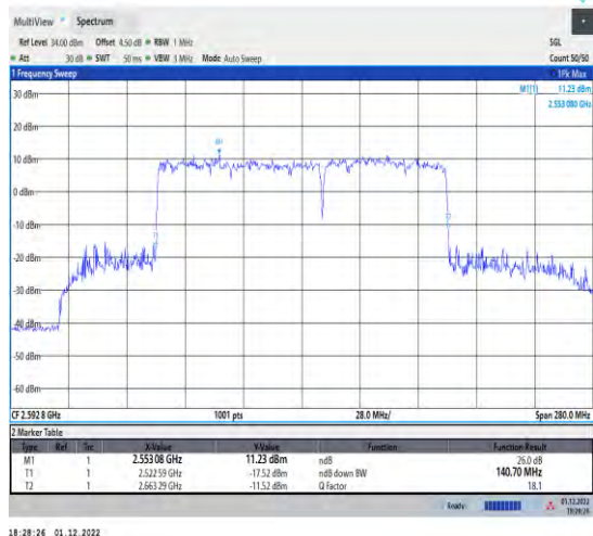
1-41-41-80+60-M-7-DFT-QPSK-Outer_Full
