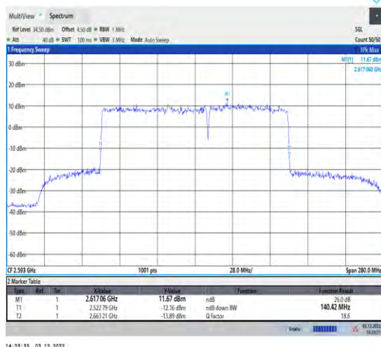
1-41-41-80+60-M-7-DFT-16QAM-Outet_Full
