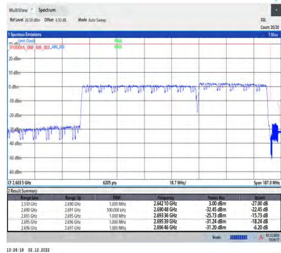
1-41-41-30-80+50-H-3-DFT-QPSK-Outer_Full
