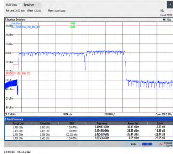
1-41-41-30-80+50-L-3-DFT-QPSK-Outer_Full
