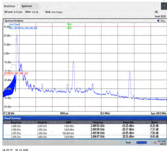
1-41-41-30-100+40-L-5-CP-QPSK-Edge_1RB_Left
