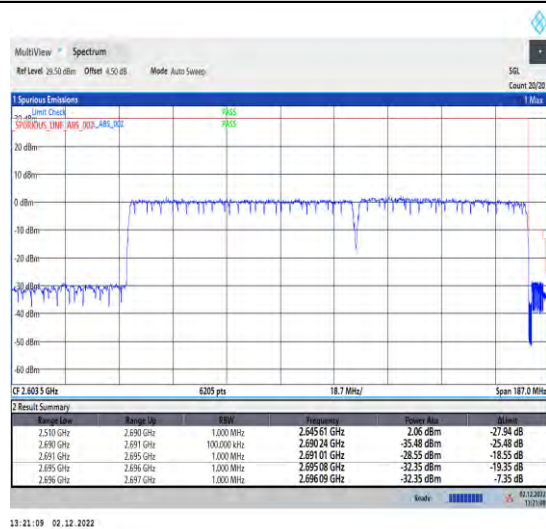
1-41-41-30-80+60-H-3-DFT-QPSK-Outer_Full
