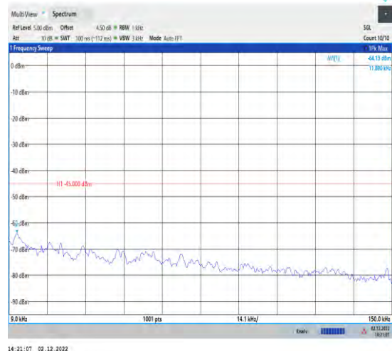
1-41-41-30-100-L-1-DFT-QPSK-Inner_1RB_Left-1@ 1-9-150
