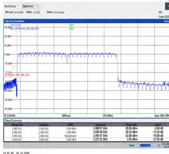
1-41-41-30-60+60-L-3-DFT-QPSK-Outer_Full
