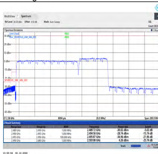
1-41-41-30-80+40-L-3-DFT-QPSK-Outer_Full
