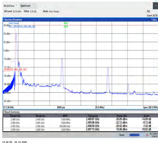
1-41-41-30-60+60-L-2-DFT-QPSK-Edge_1RB_Left
