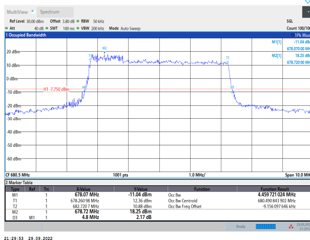
Band71-5MHz-QPSK-133297-25RB#0
