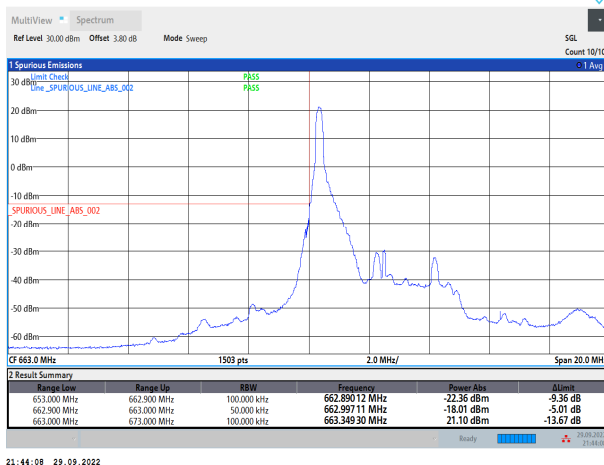
Band71-5MHz-QPSK-133147-25RB#0
