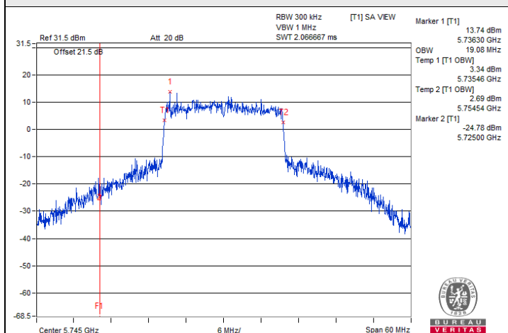
802.11be (EHT20) CDD / Chain 2 : CH 149
