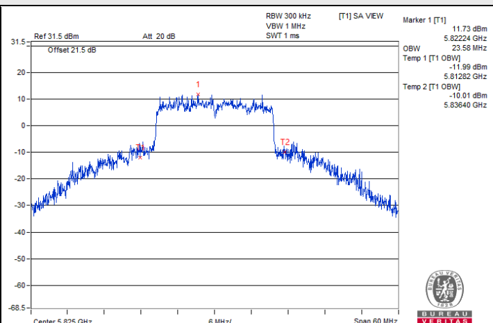
802.11be (EHT20) CDD / Chain 3 : CH 165
