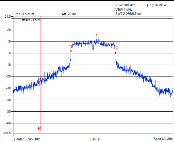
802.11a CDD / Chain 3 : CH 149
