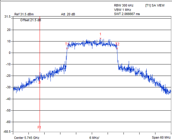
802.11be (EHT20) CDD / Chain 1 : CH 149
