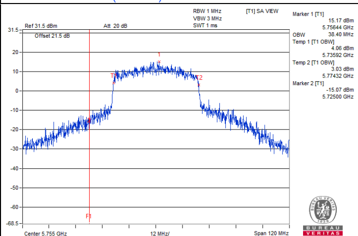
802.11be (EHT40) CDD / Chain 1 : CH 151
