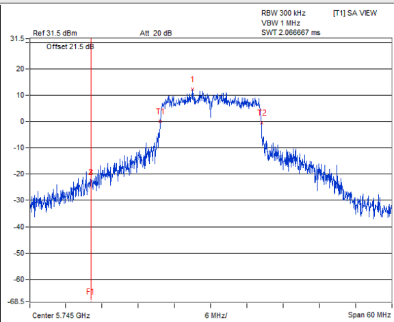
802.11a CDD / Chain 1 : CH 149
