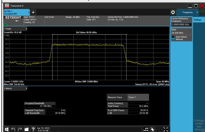
BPSK CH 633334 (3500.01 MHz)
