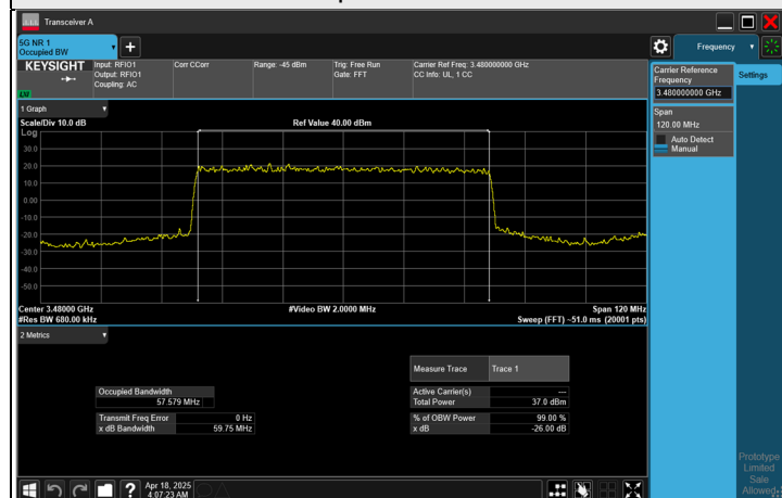
BPSK CH 632000 (3480 MHz)
