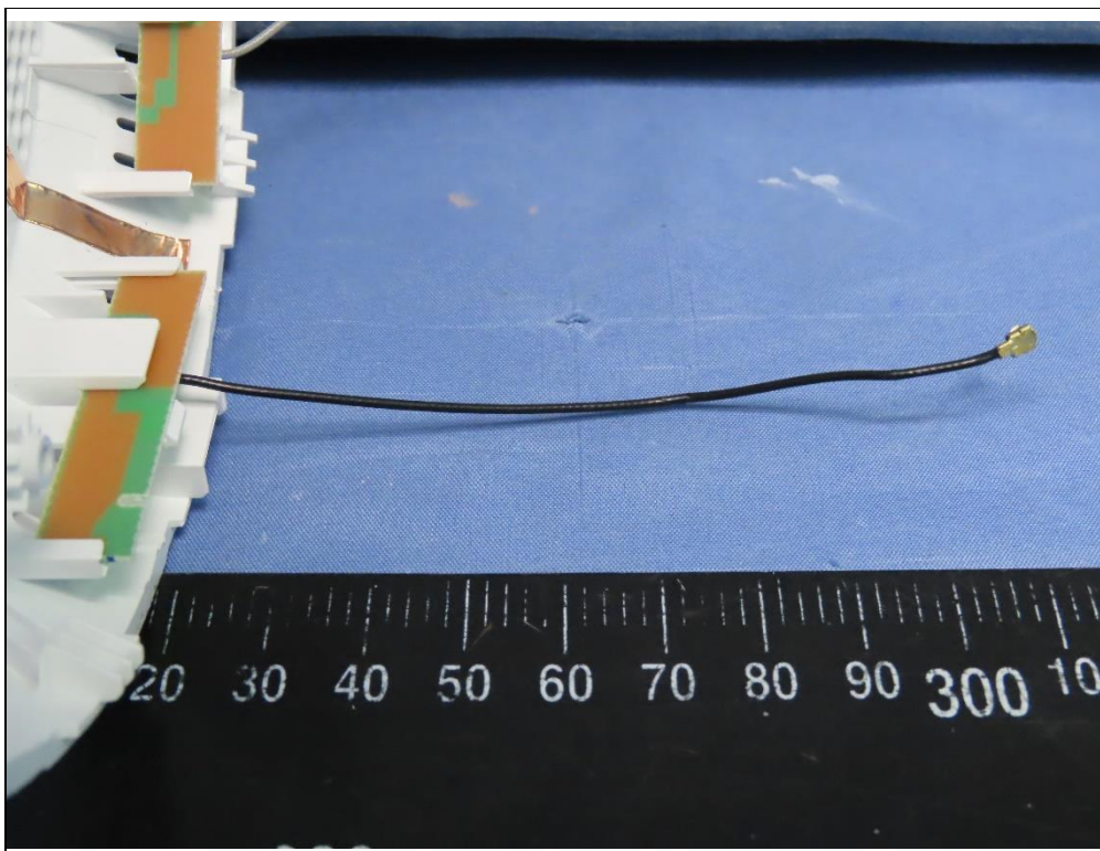
Antenna 1 (Brand: LITE , Model: 520101-7002-23R)
