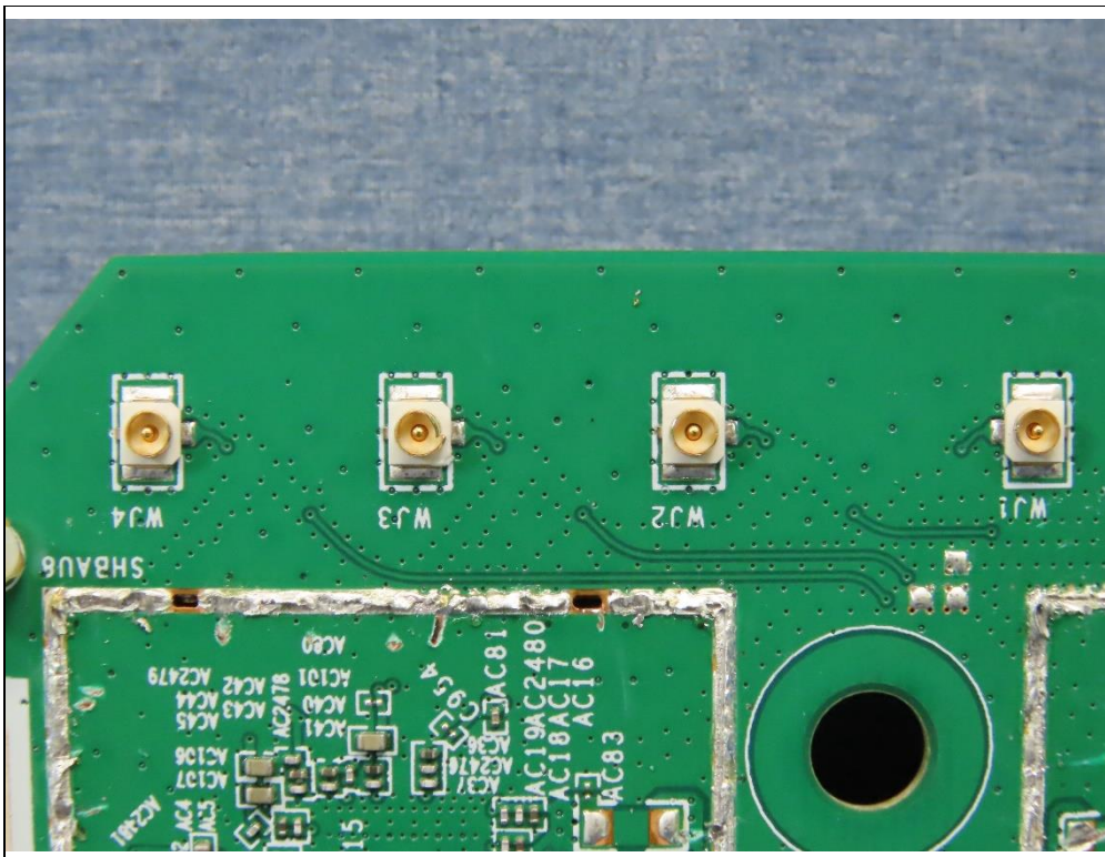
Antenna 0 (Brand: LITE , Model: 520101-7001-23R)
