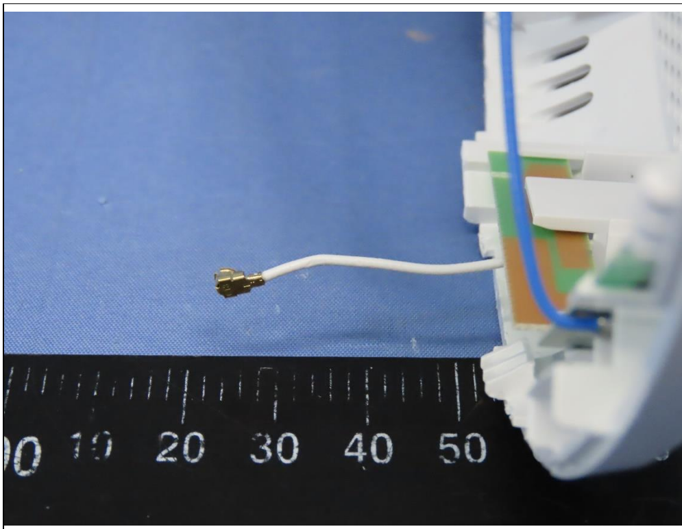
Antenna 3 (Brand: LITE , Model: 520101-7003-23R)
