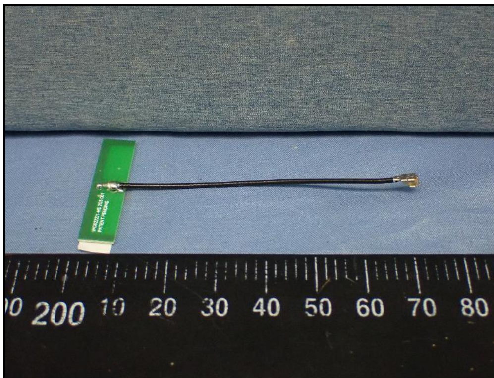
Ant. Set 1 (Chain 1 / 2G5 001)
