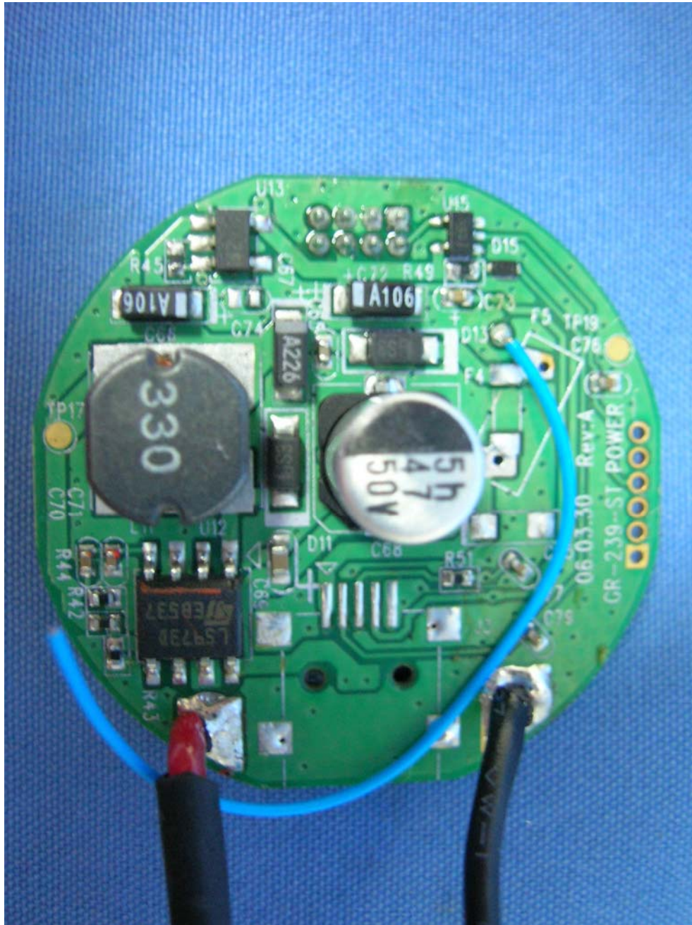
(12) EUT Photo
