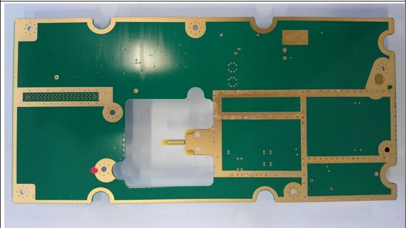
HALO RX PCBA
