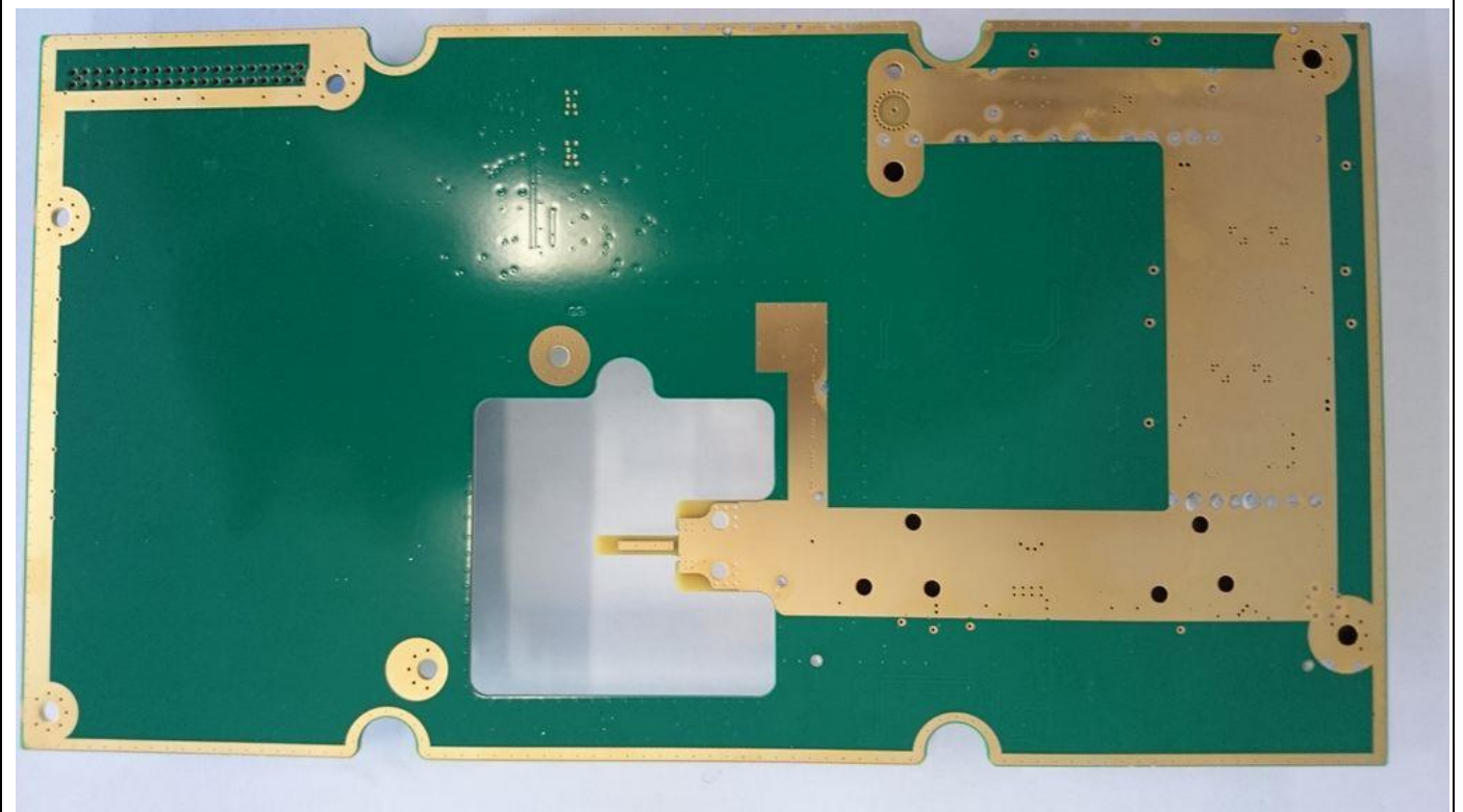
HALO PA PCBA
