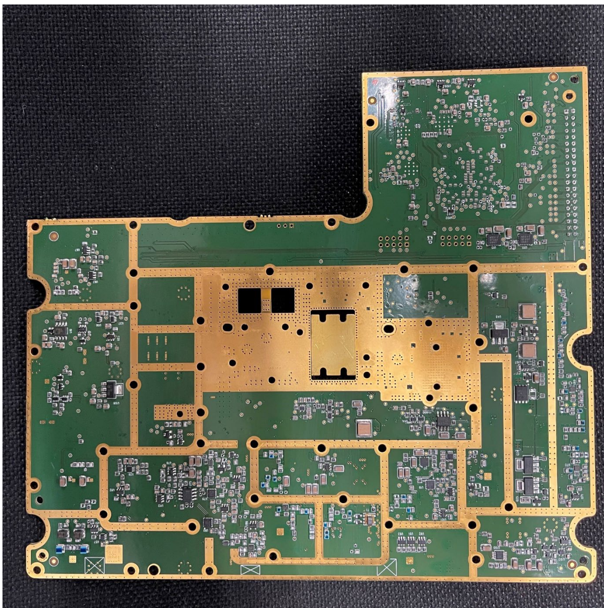
RF PCBA
