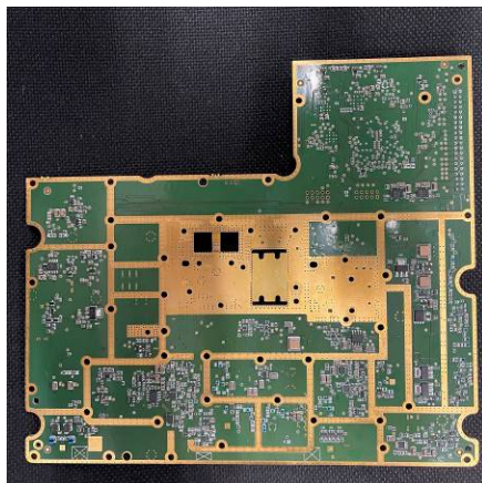
RF PCBA - top
