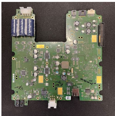
CPU PCBA - top
