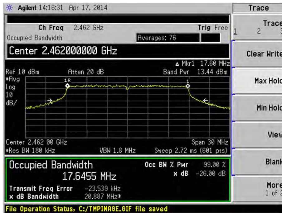
802.11 n-HT20 (Channel 11)
