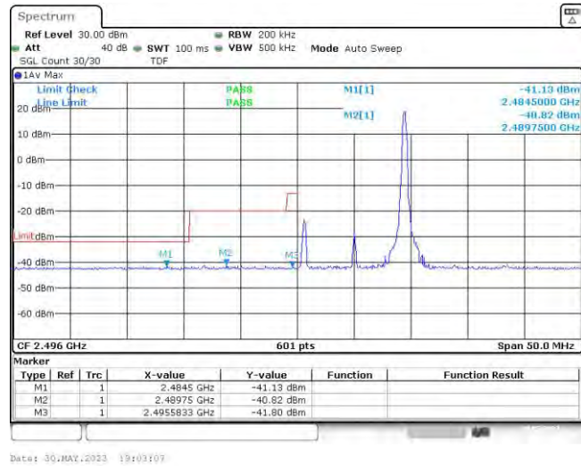
Band41-10MHz-QPSK-39700-50RB#0
