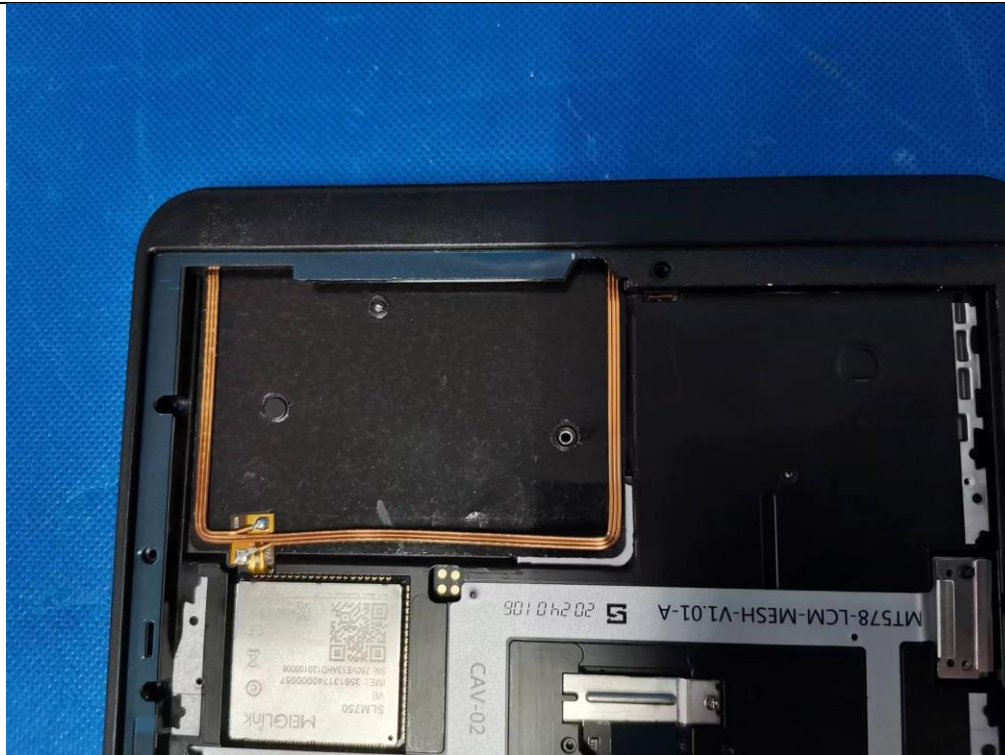
EUT Photo(8) - NFC Antenna
