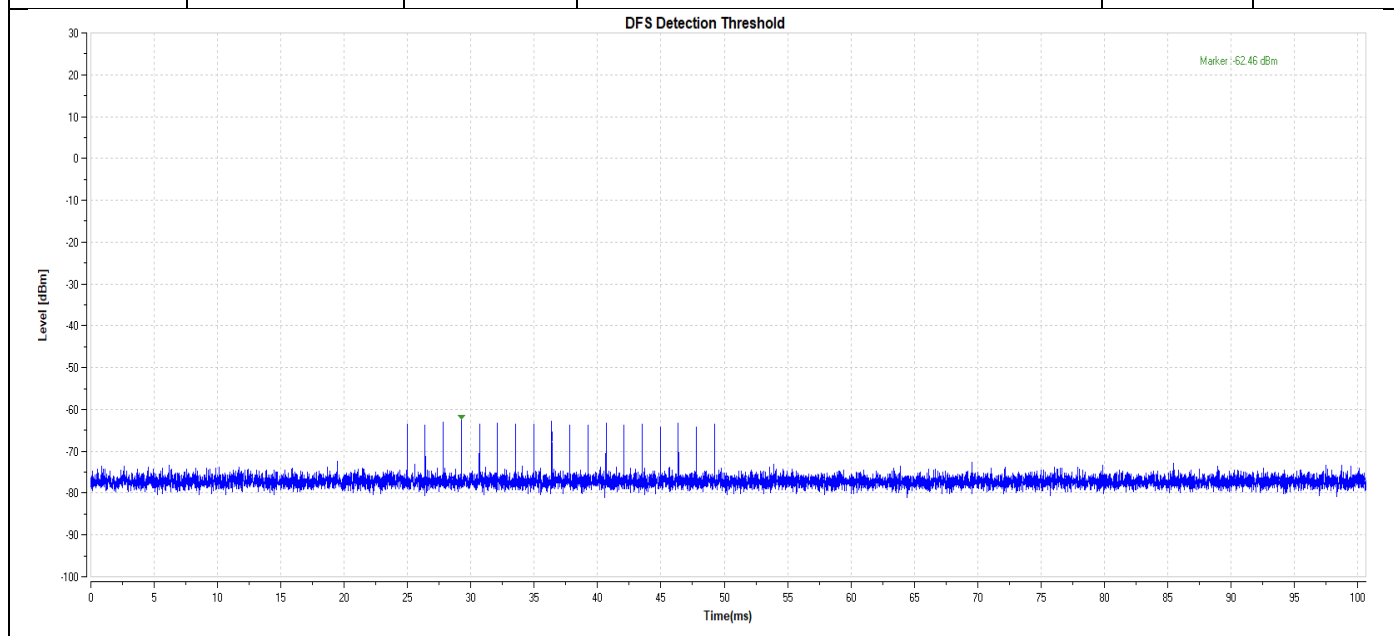
11AC80SISO-5290-Type0-PASS
