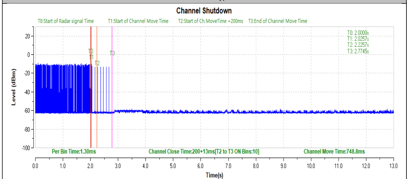
11AC80SISO-5290-Type0-PASS
