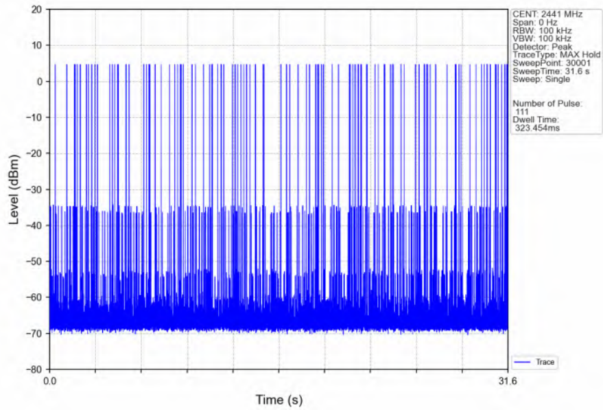
Pi/4DQPSK_2DH5_HOPP_Ant1_NTNV
