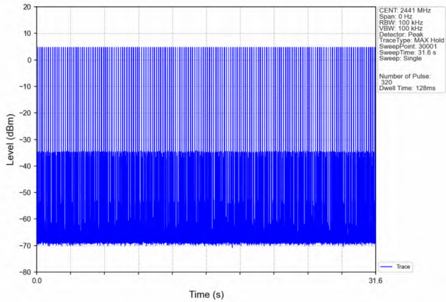
Pi/4DQPSK_2DH1_HOPP_Ant1_NTNV
