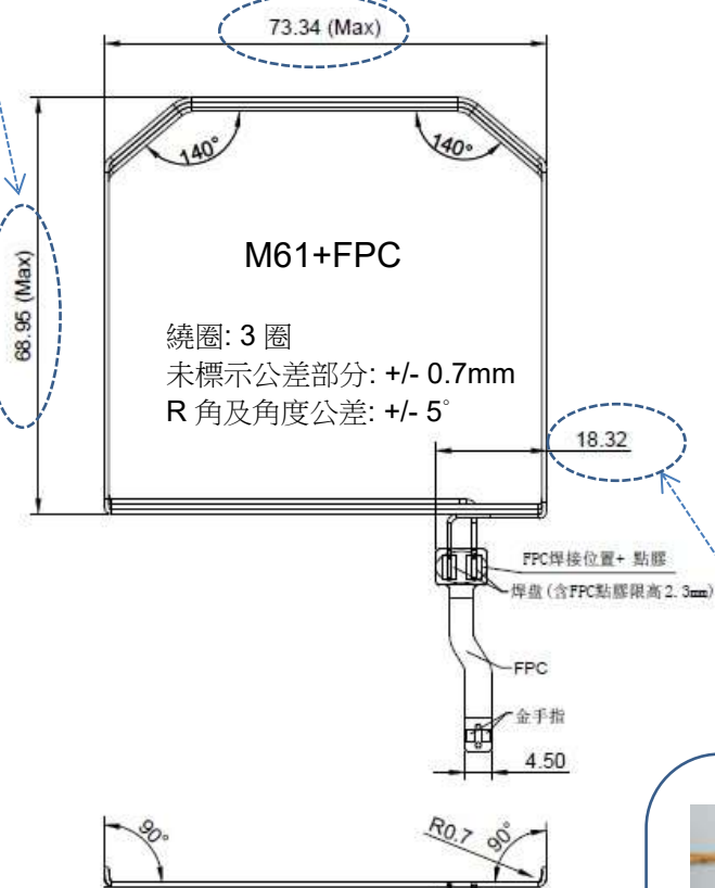
尺寸 A
