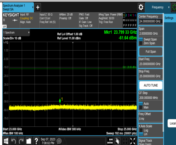
BLE_2M_Ant1_2480_23000~25000
