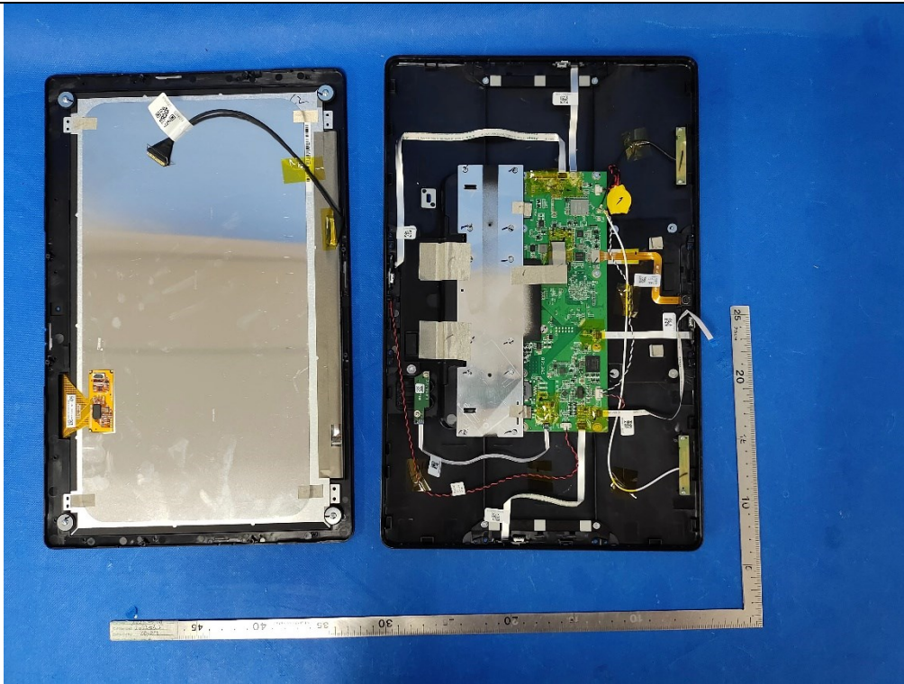
(16) EUT Photo ( ESY15I4 )
