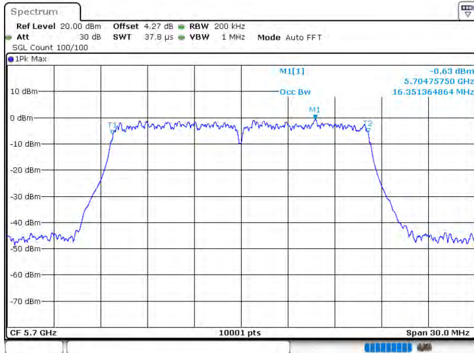
OBW NVNT a 5700MHz Ant0
