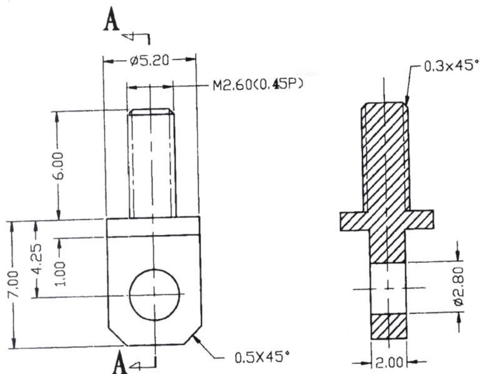
SEC A-A
