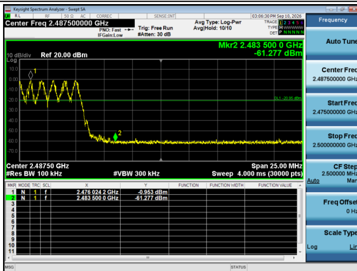
DH5_Ant1_Hop_High
