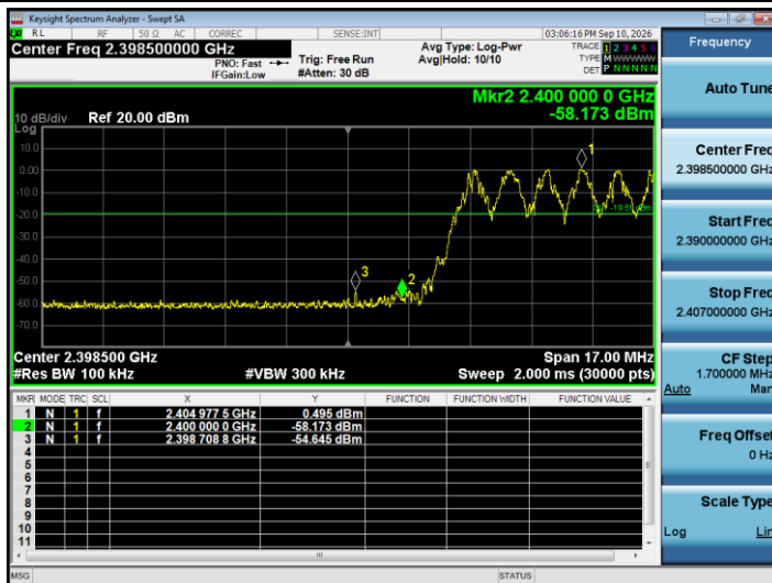
DH5_Ant1_Hop_Low
