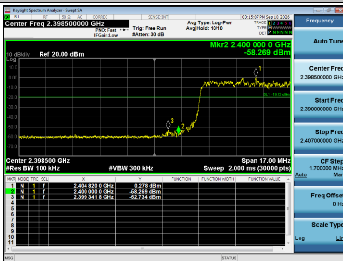
2DH5_Ant1_Hop_Low
