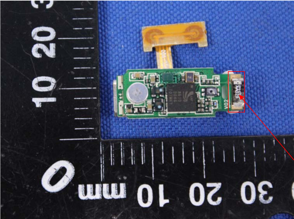
Antenna
