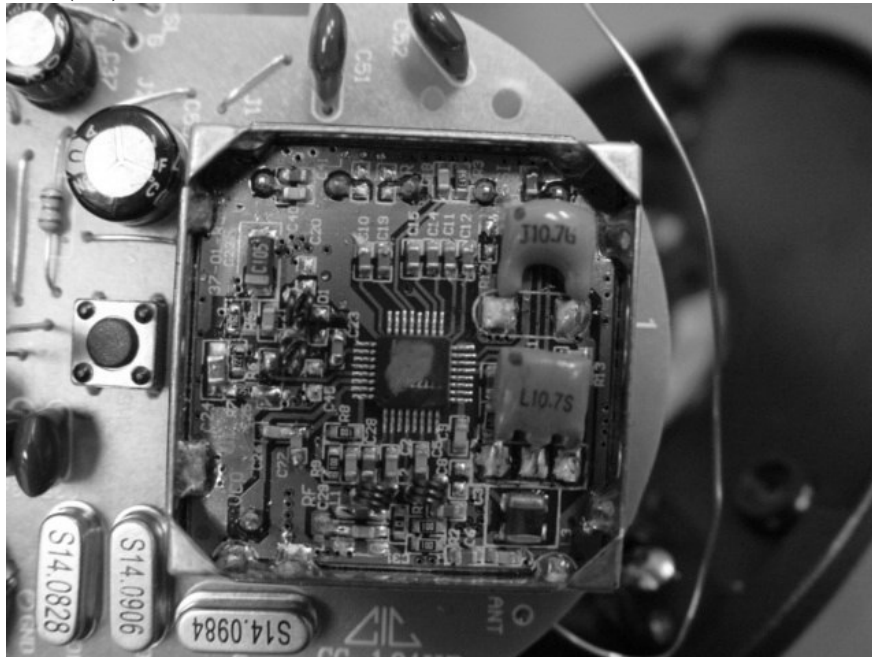
UHF module (Rx)
