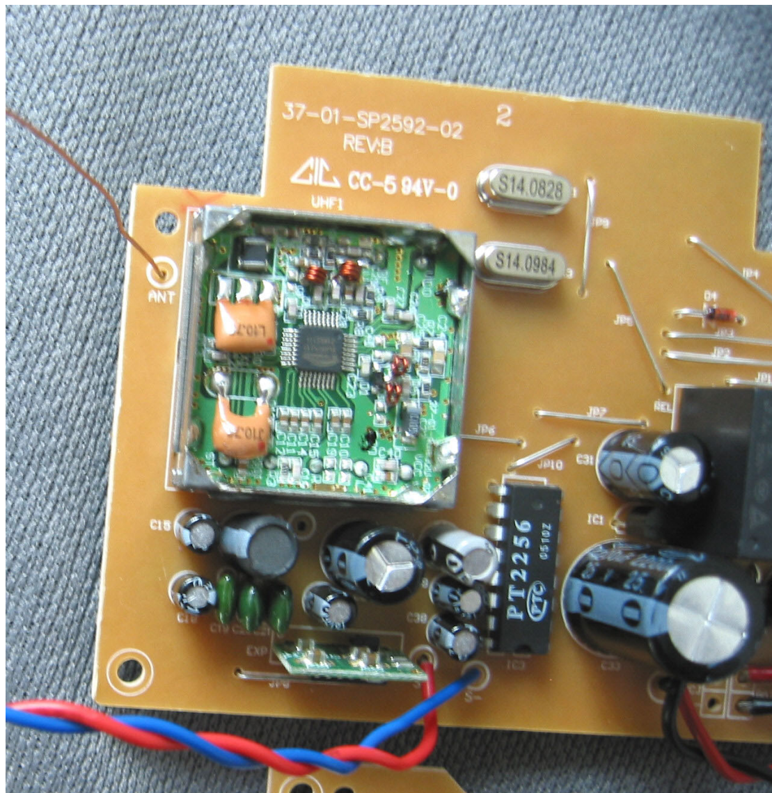
UHF module(RX)
