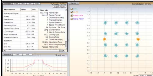
5MHz, 16QAM
