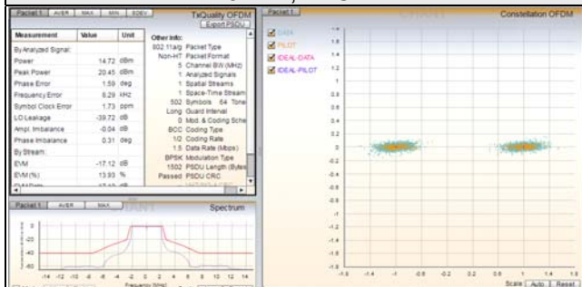
5MHz, BPSK
