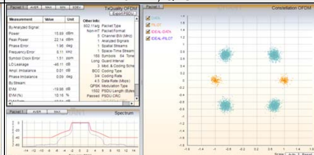
5MHz, QPSK
