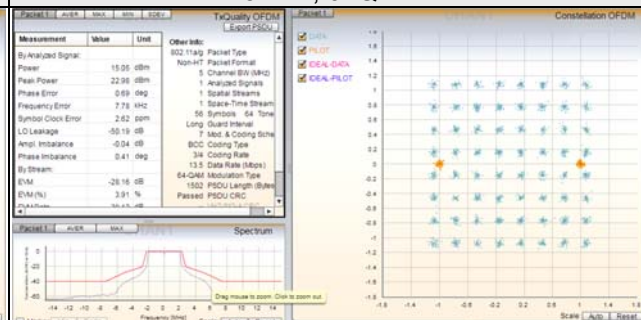
5MHz, 64QAM
