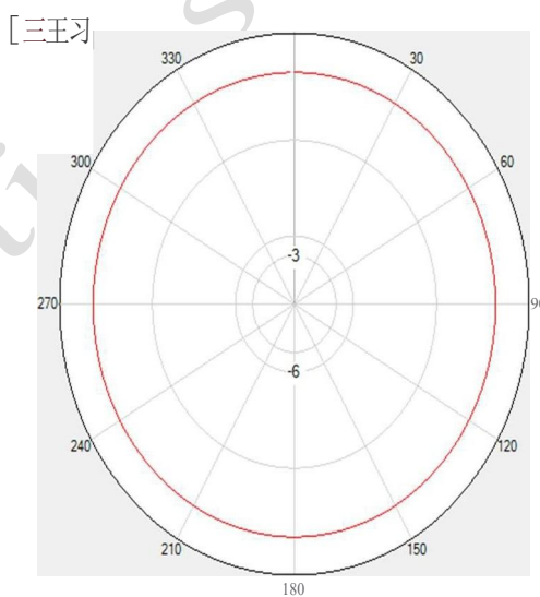
HTheta=0
