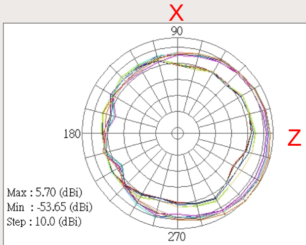
E1 plane
