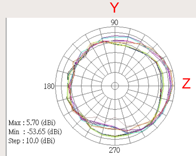
E2 plane
