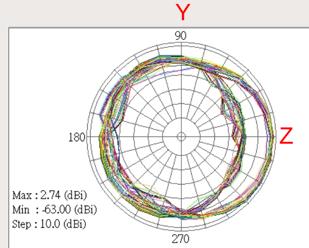
E2 plane
