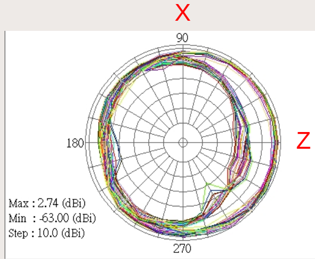
E1 plane
