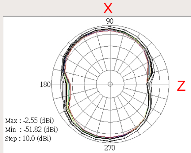
E1 plane
