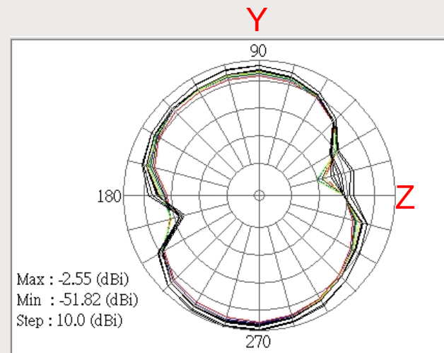
E2 plane
