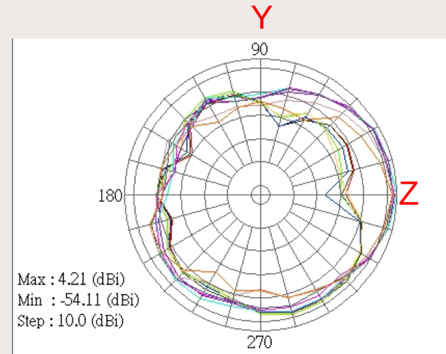
E2 plane
