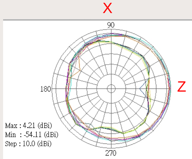
E1 plane
