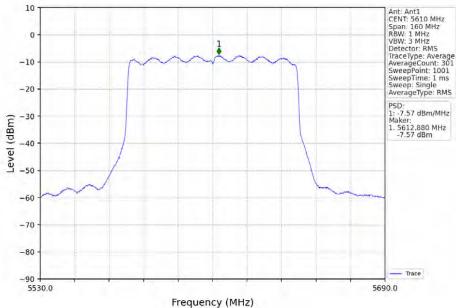
802.11ax(HEW80)_HCH_5610MHz_RU996_Left_Ant1_NTNV
