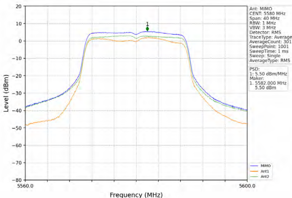
802.11n(HT20)_MCH_5580MHz_MIMO_NTNV
