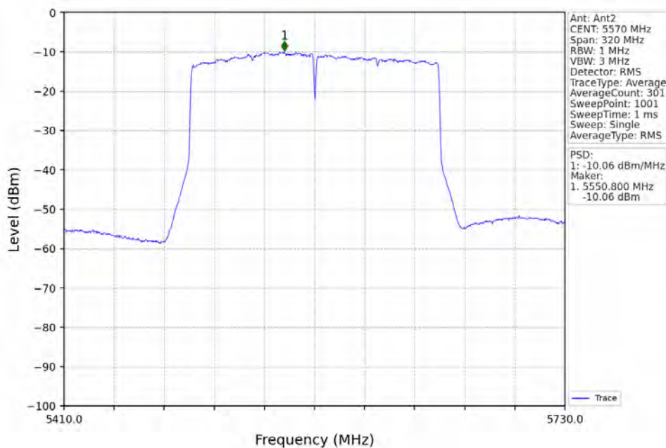
802.11ax(HEW160)_MCH_5570MHz_2xRU996_Left_Ant2_NTNV
