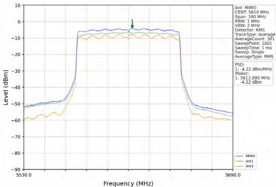
802.11ax(HEW80)_HCH_5610MHz_RU996_Left_MIMO_NTNV
