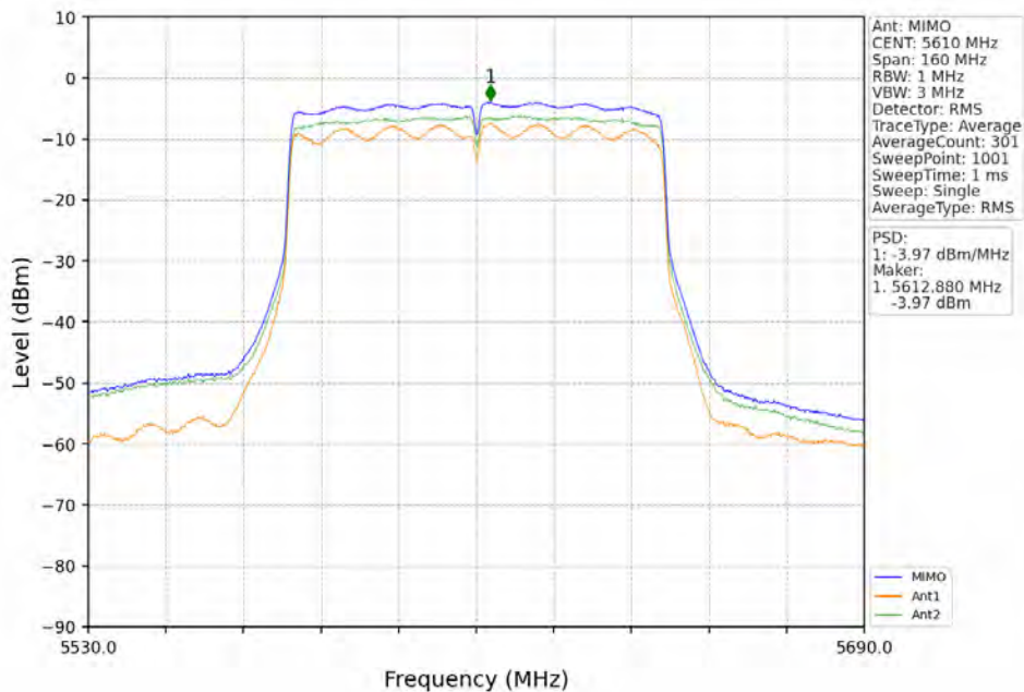
802.11ac(VHT80)_HCH_5610MHz_MIMO_NTNV
