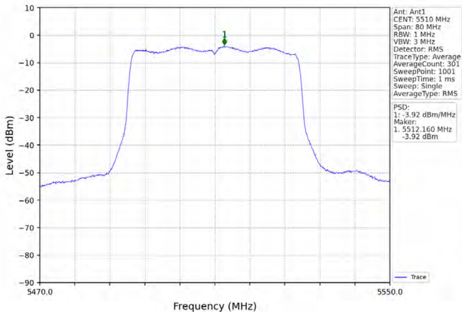
802.11ax(HEW40)_LCH_5510MHz_RU484_Left_Ant1_NTNV
