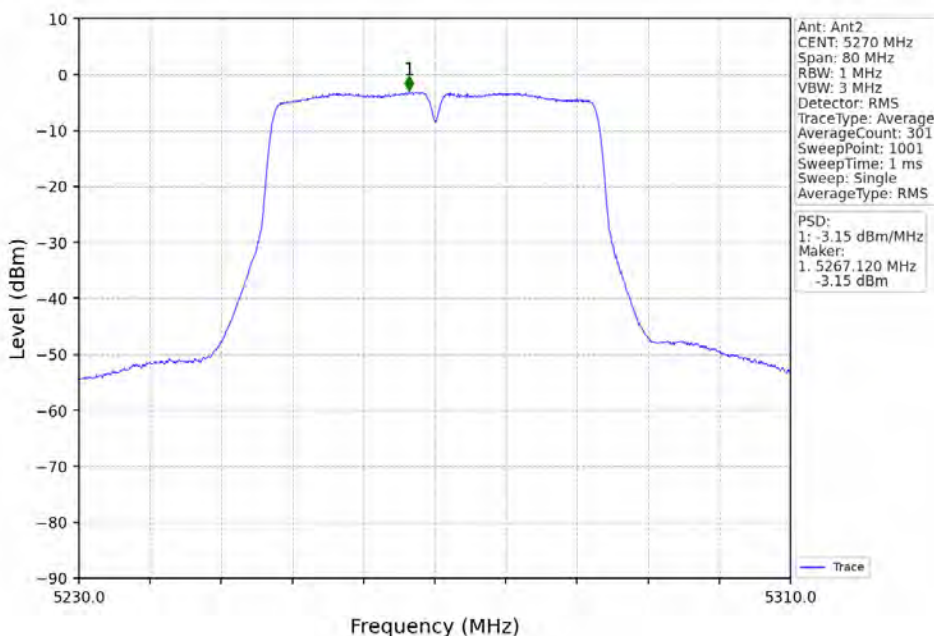
802.11n(HT40)_LCH_5270MHz_MIMO_NTNV
