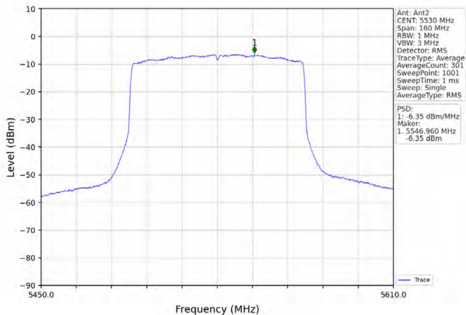
802.11ax(HEW80)_LCH_5530MHz_RU996_Left_Ant2_NTNV
