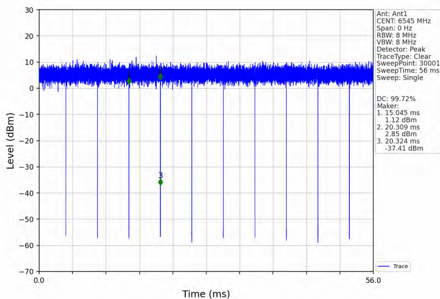
802.11ax(HEW80)_HCH_6545MHz_RU996_Left_Ant1_NTNV
