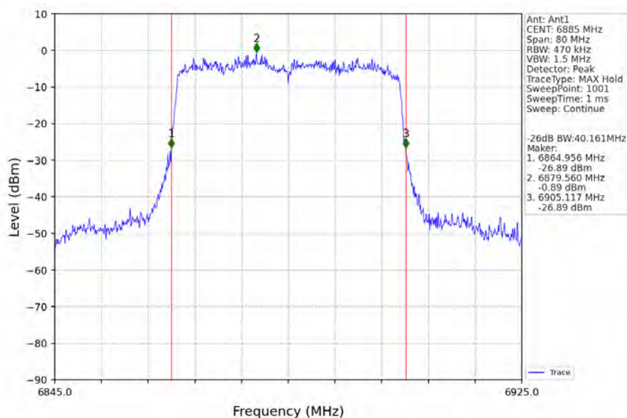
802.11ax(HEW40)_HCH_6885MHz_RU484_Left_Ant1_NTNV
