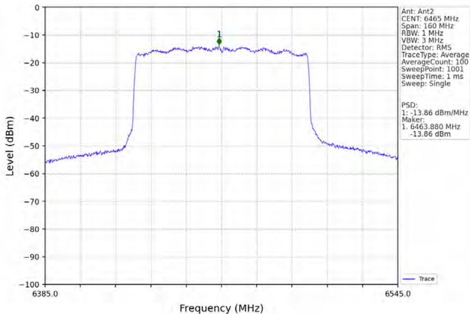
802.11ax(HEW80)_LCH_6465MHz_RU996_Left_MIMO_NTNV
