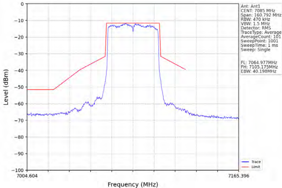
802.11ax(HEW40)_HCH_7085MHz_RU484_Left_Ant1_NTNV
