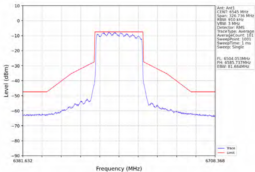
802.11ax(HEW80)_HCH_6545MHz_RU996_Left_Ant1_NTNV
