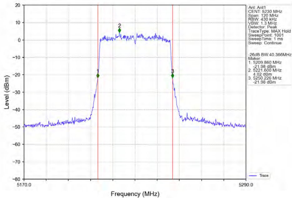
802.11ax(HEW40)_HCH_5230MHz_RU484_Left_Ant5_NTNV
