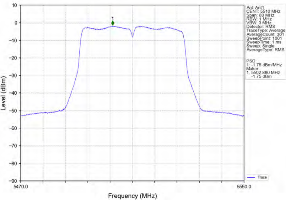
802.11n(HT40)_LCH_5510MHz_Ant1_NTNV
