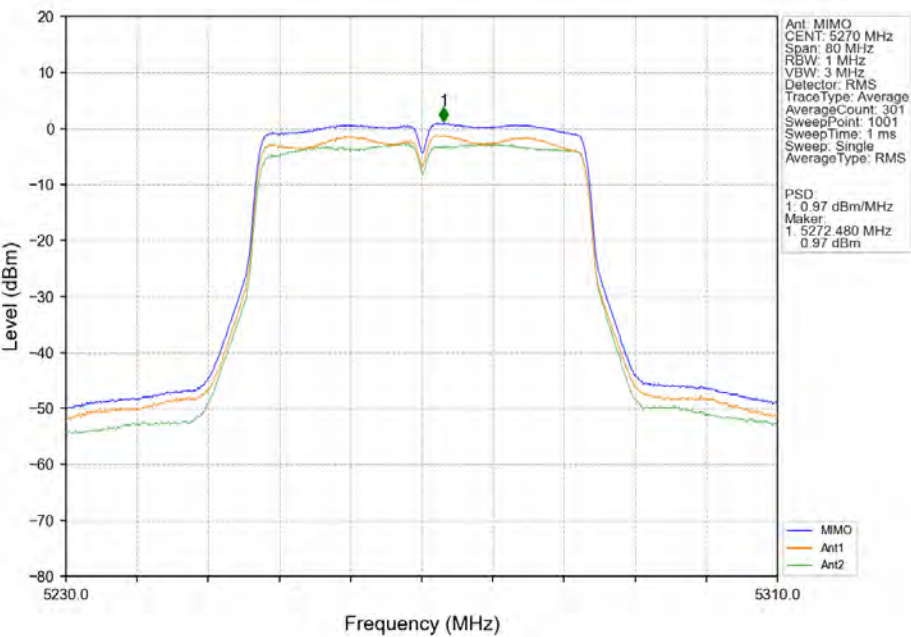
802.11n(HT40)_LCH_5270MHz_MIMO_NTNV
