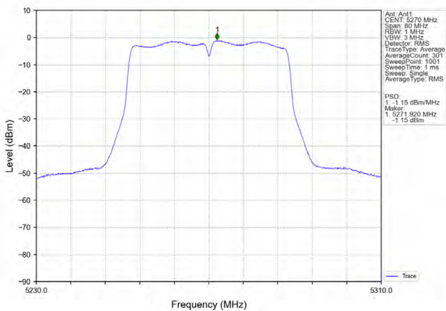
802.11n(HT40)_LCH_5270MHz_Ant1_NTNV
