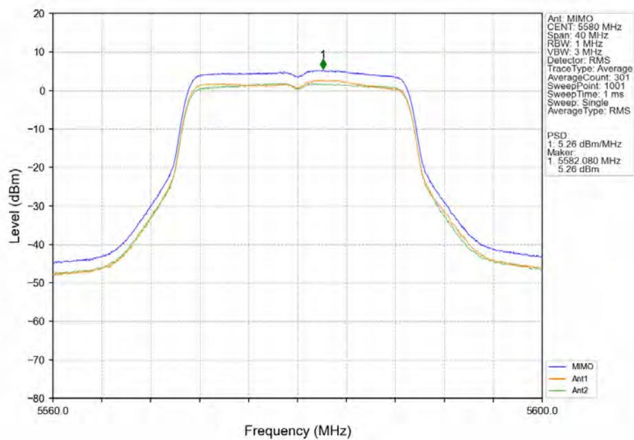
802.11n(HT20)_MCH_5580MHz_MIMO_NTNV
