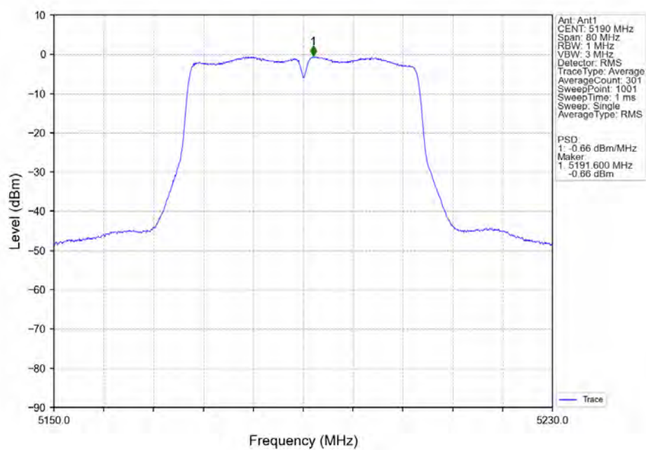
802.11n(HT40)_LCH_5190MHz_Ant1_NTNV
