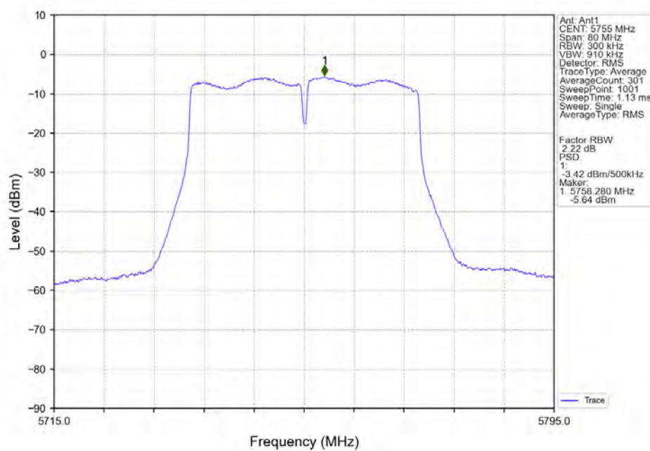
802.11n(HT40)_LCH_5755MHz_Ant1_NTNV
