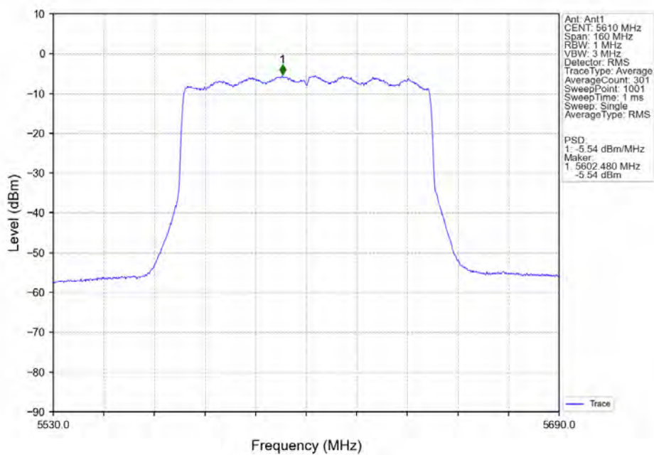
802.11ax(HEW80)_HCH_5610MHz_RU996_Left_Ant1_NTNV
