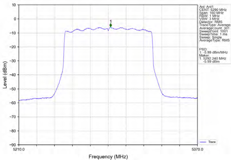
802.11ax(HEW80)_MCH_5290MHz_RU996_Left_Ant1_NTNV
