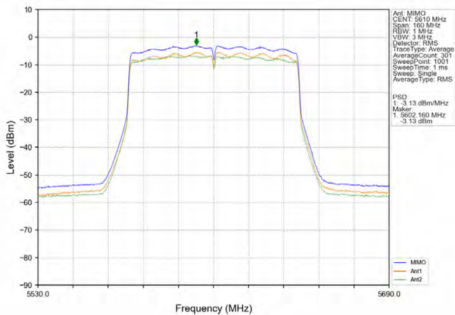
802.11ac(VHT80)_HCH_5610MHz_MIMO_NTNV
