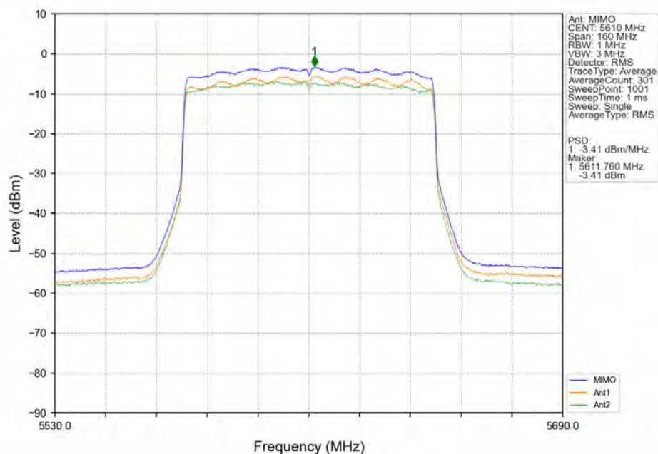
802.11ax(HEW80)_HCH_5610MHz_RU996_Left_MIMO_NTNV
