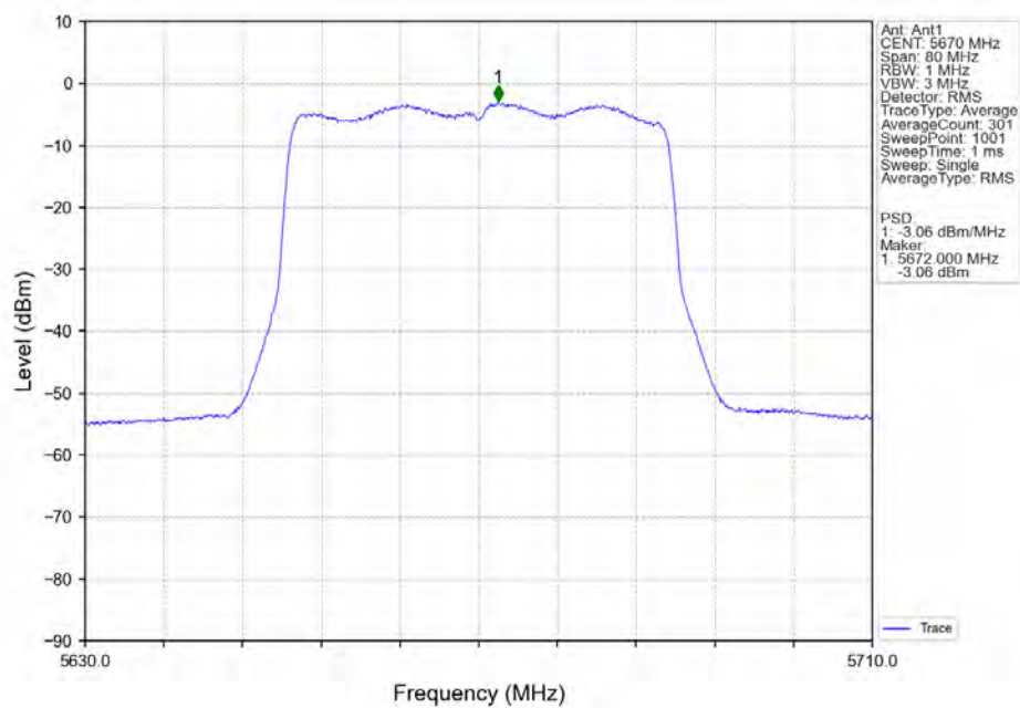
802.11ax(HEW40)_HCH_5670MHz_RU484_Left_Ant1_NTNV
