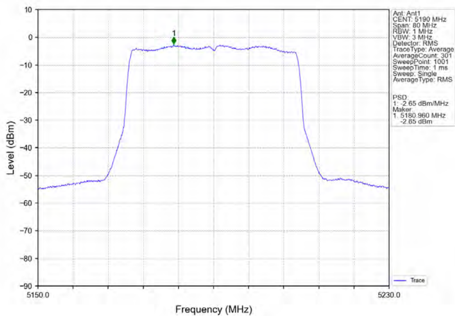
802.11ax(HEW40)_LCH_5190MHz_RU484_Left_Ant1_NTNV
