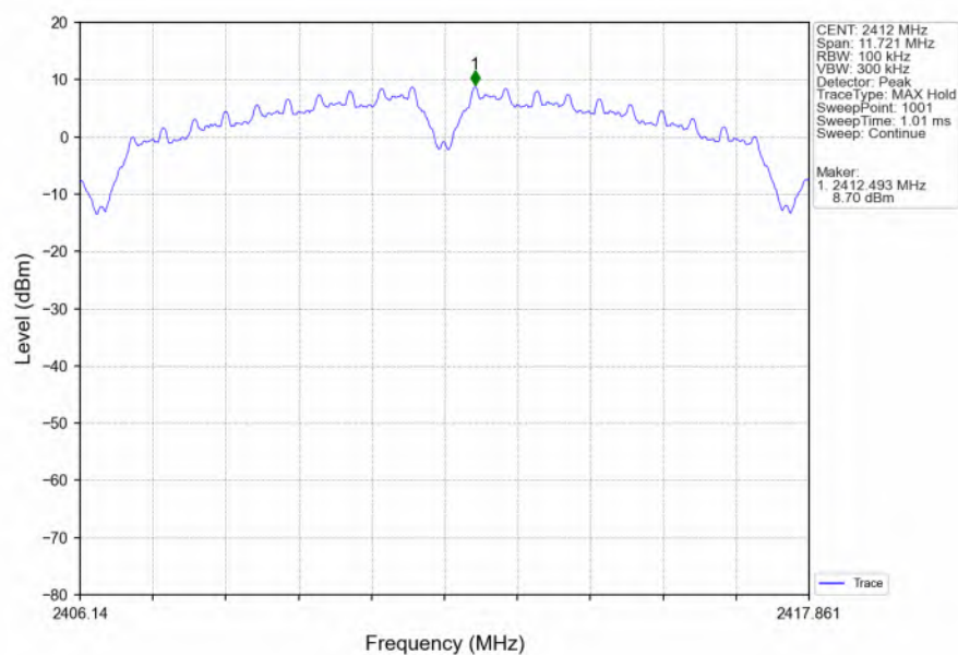
802.11b_LCH_2412MHz_Ant6 (SISO)_NTNV
