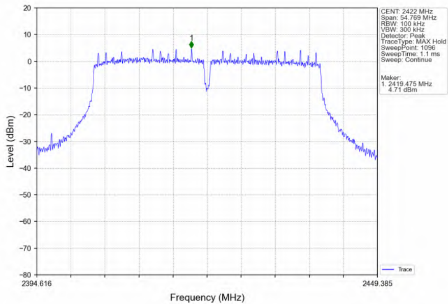
802.11n(HT40)_LCH_2422MHz_Ant6 (MIMO)_NTNV
