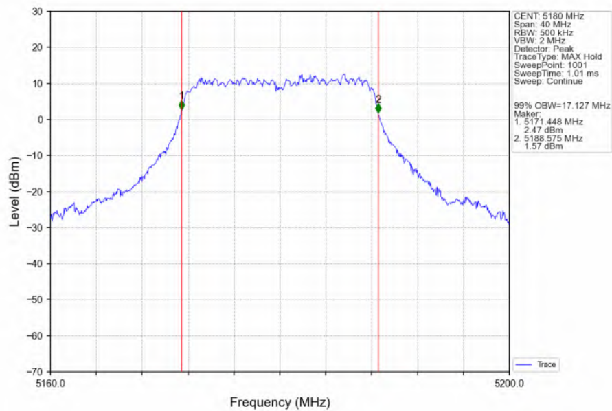
802.11a_LCH_5180MHz_Ant6_NTNV
