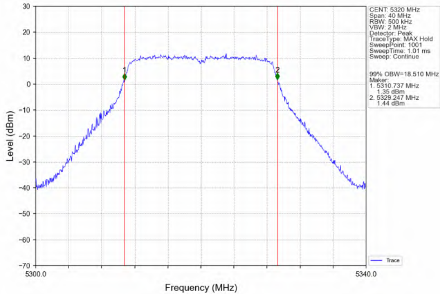
802.11n(HT20)_HCH_5320MHz_Ant6_NTNV
