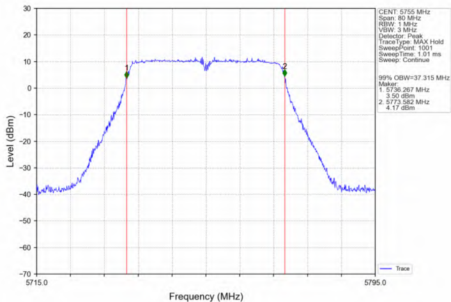
802.11ac(VHT40)_LCH_5755MHz_Ant6_NTNV
