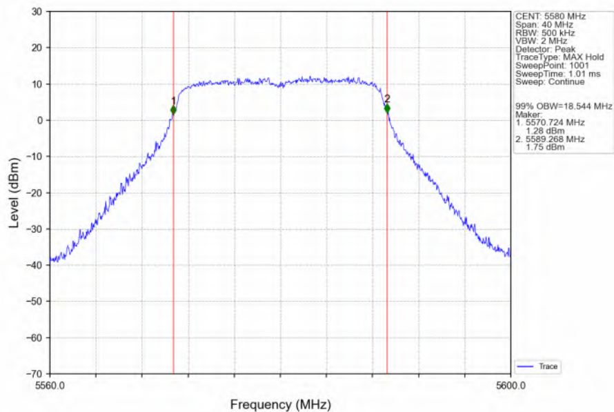
802.11n(HT20)_MCH_5580MHz_Ant6_NTNV
