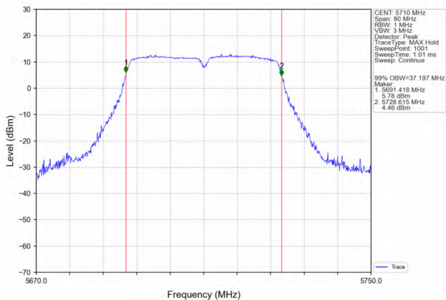
802.11n(HT40)_HCH_5710MHz_Ant6_NTNV
