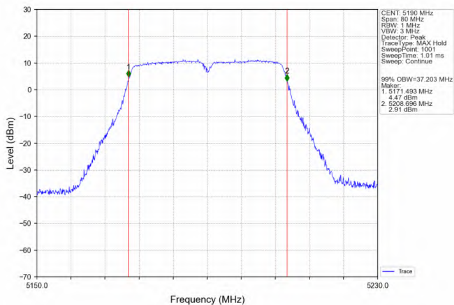
802.11n(HT40)_LCH_5190MHz_Ant6_NTNV
