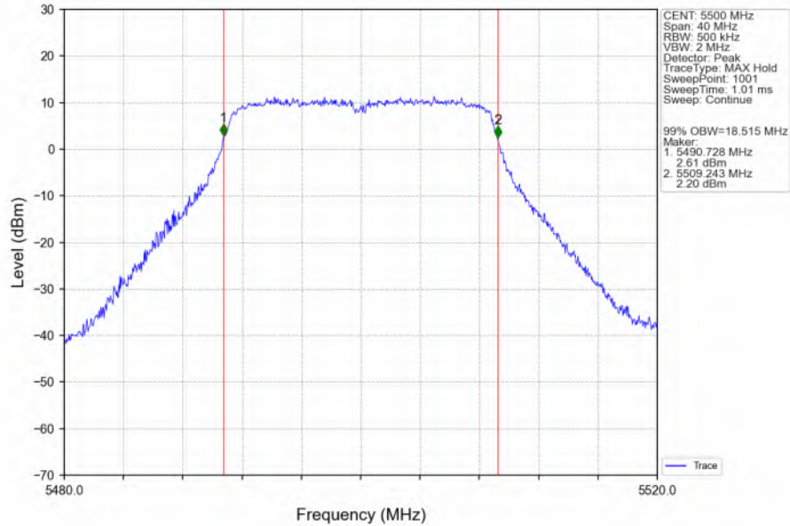
802.11n(HT20)_LCH_5500MHz_Ant6_NTNV
