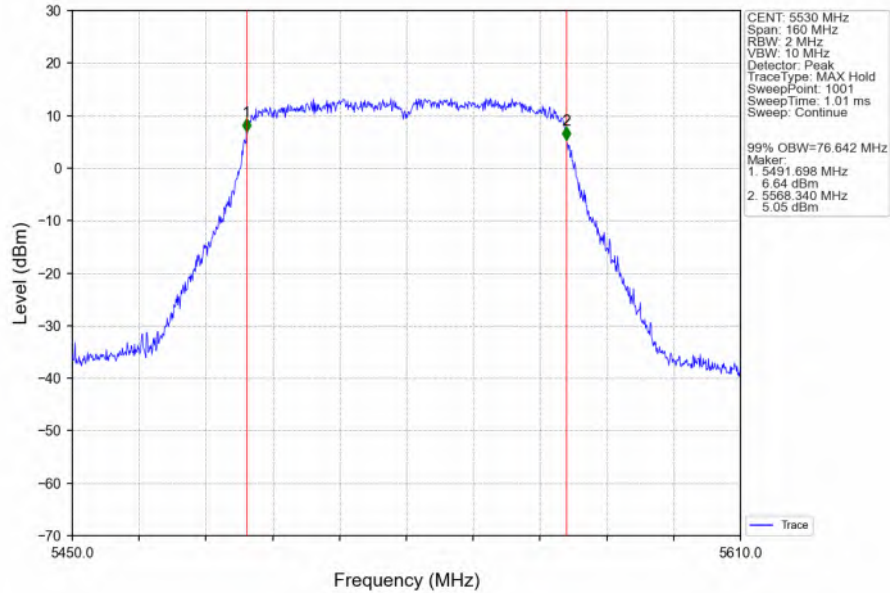
802.11ac(VHT80)_LCH_5530MHz_Ant6_NTNV
