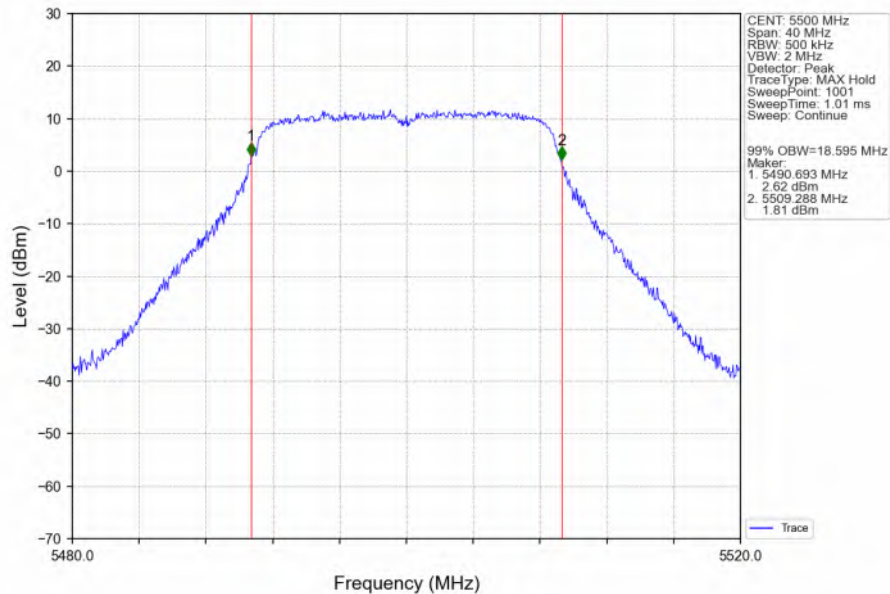
802.11ac(VHT20)_LCH_5500MHz_Ant6_NTNV
