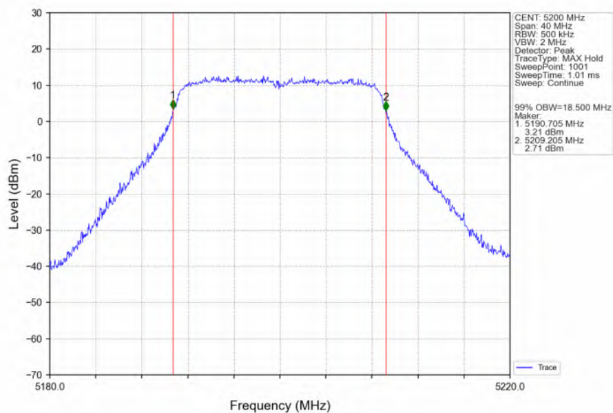
802.11n(HT20)_MCH_5200MHz_Ant6_NTNV
