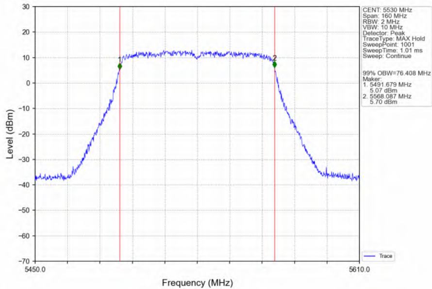
802.11ac(VHT80)_LCH_5530MHz_Ant6_NTNV
