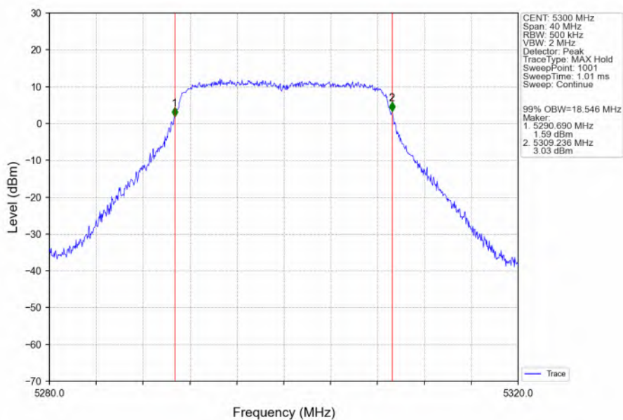
802.11n(HT20)_MCH_5300MHz_Ant6_NTNV
