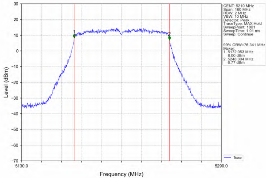
802.11ac(VHT80)_MCH_5210MHz_Ant6_NTNV
