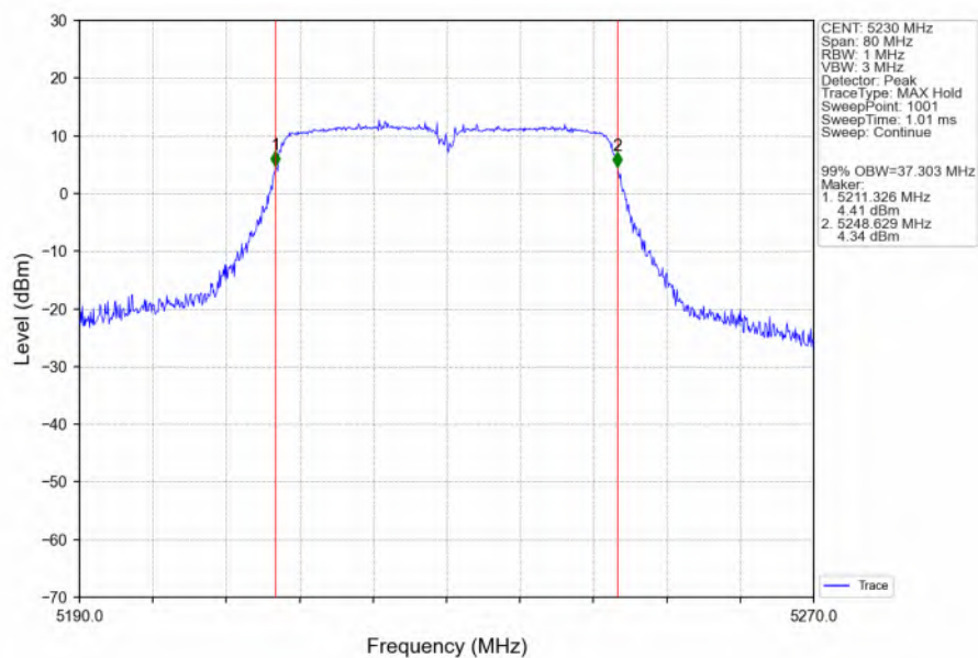
802.11ac(VHT40)_HCH_5230MHz_Ant6_NTNV
