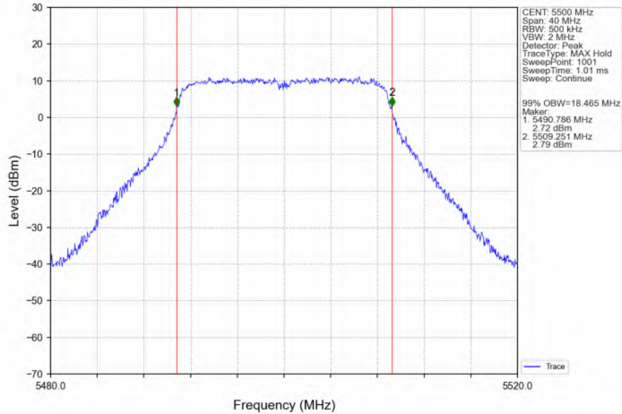
802.11ac(VHT20)_LCH_5500MHz_Ant6_NTNV
