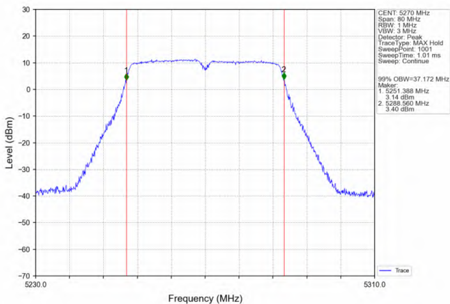
802.11n(HT40)_LCH_5270MHz_Ant6_NTNV
