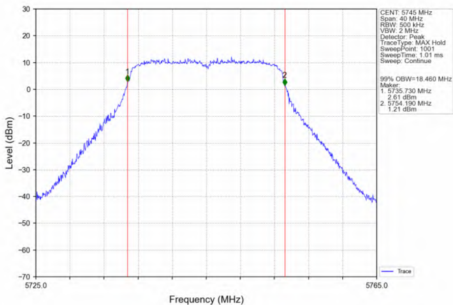
802.11n(HT20)_LCH_5745MHz_Ant6_NTNV
