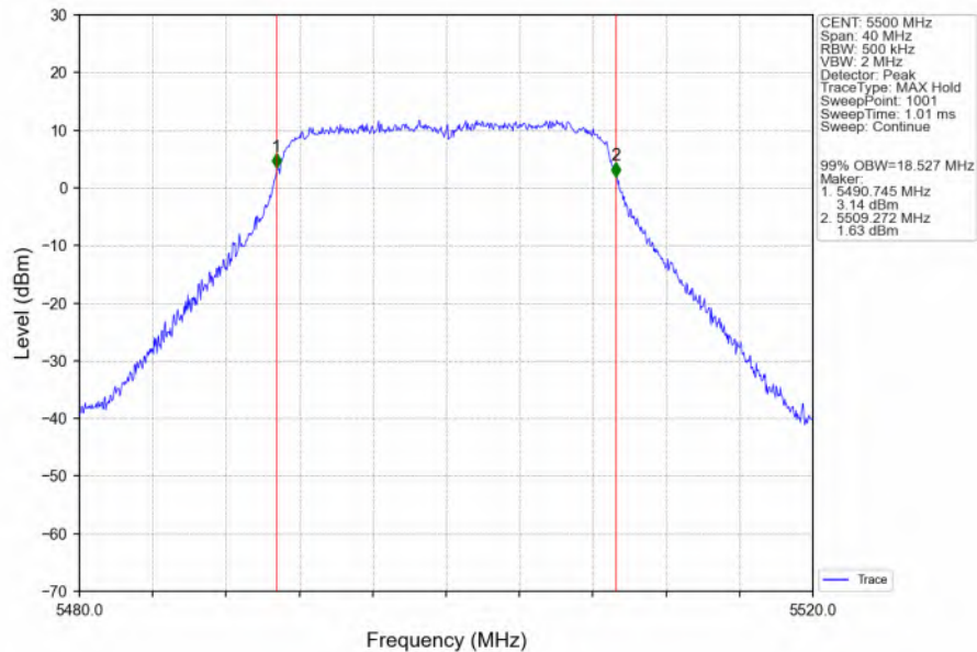
802.11n(HT20)_LCH_5500MHz_Ant6_NTNV
