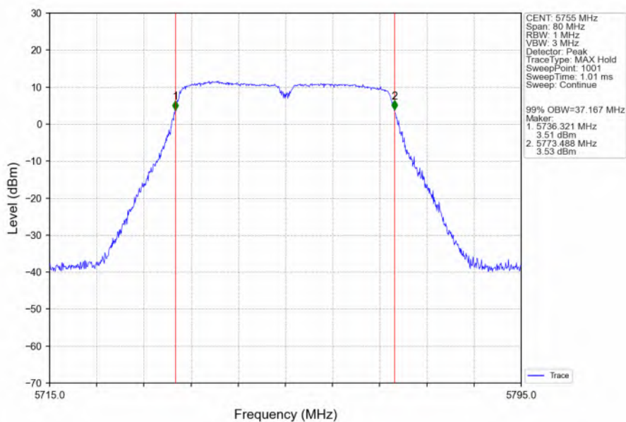
802.11n(HT40)_LCH_5755MHz_Ant6_NTNV
