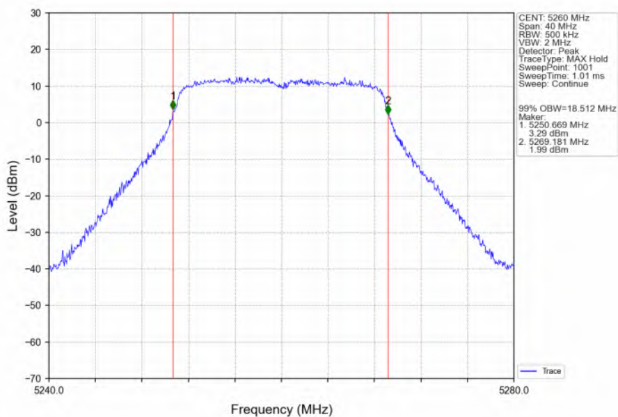
802.11n(HT20)_LCH_5260MHz_Ant6_NTNV
