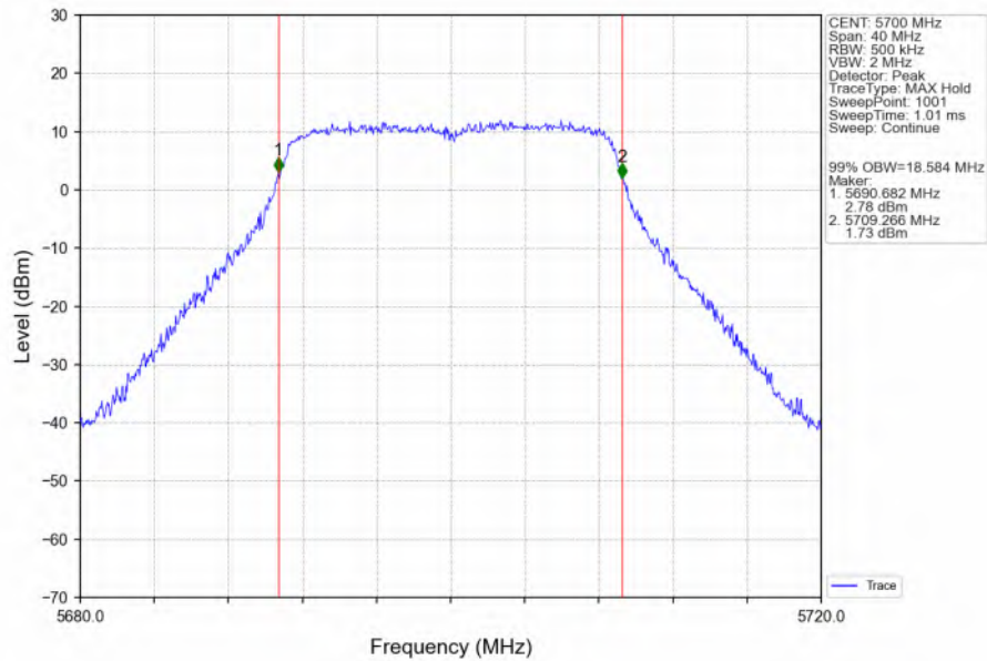
802.11n(HT20)_HCH_5700MHz_Ant6_NTNV
