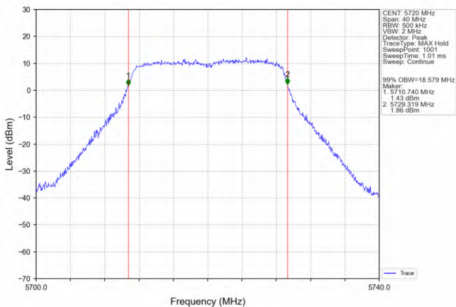
802.11n(HT20)_HCH_5720MHz_Ant6_NTNV
