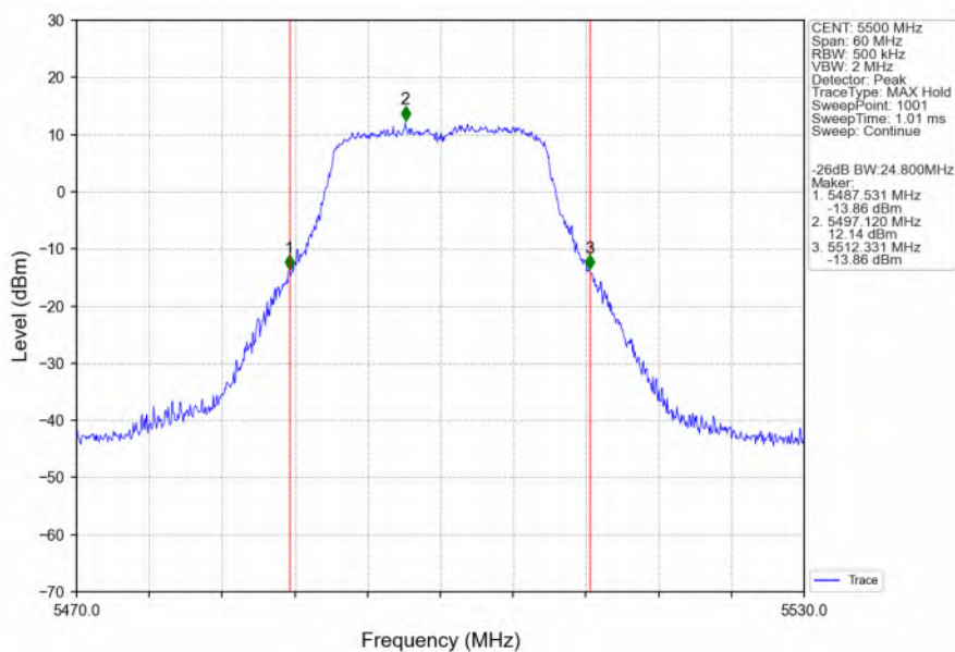
802.11n(HT20)_LCH_5500MHz_Ant6_NTNV
