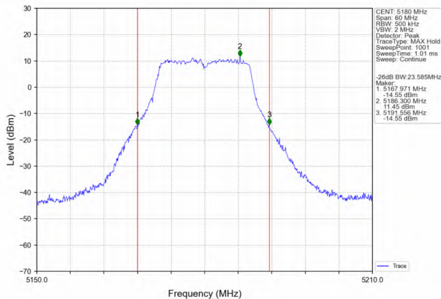
802.11a_LCH_5180MHz_Ant6_NTNV
