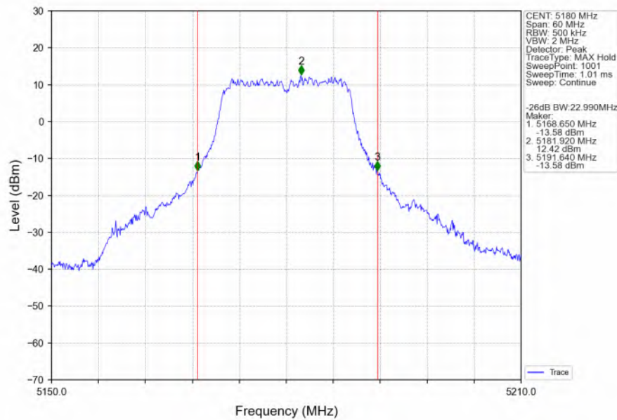
802.11a_LCH_5180MHz_Ant6_NTNV
