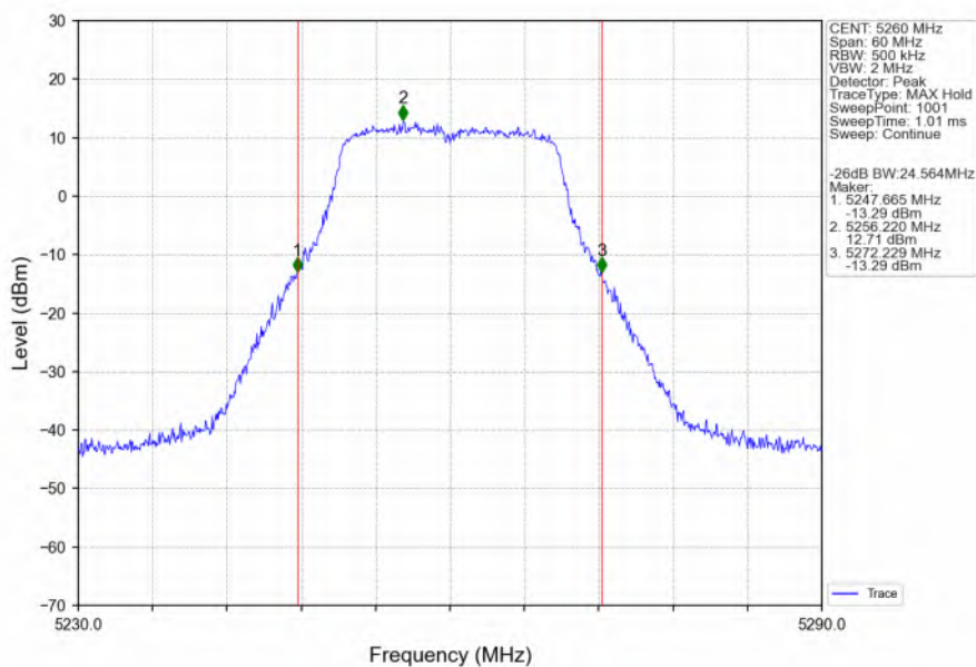
802.11n(HT20)_LCH_5260MHz_Ant6_NTNV
