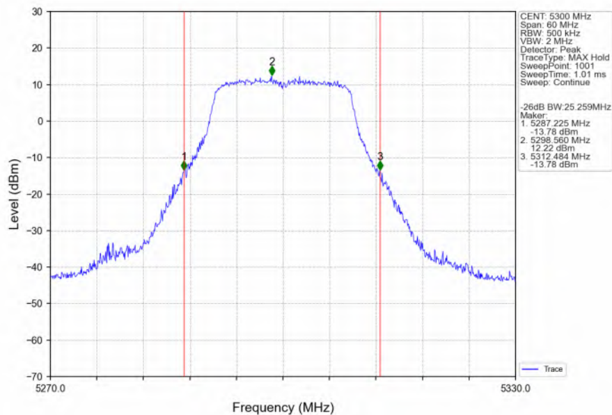
802.11n(HT20)_MCH_5300MHz_Ant6_NTNV
