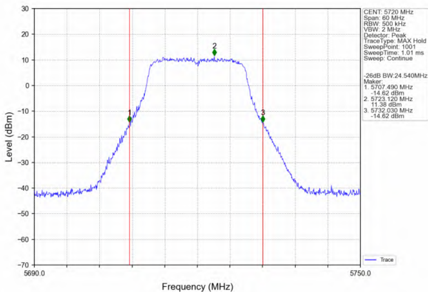
802.11n(HT20)_HCH_5720MHz_Ant6_NTNV
