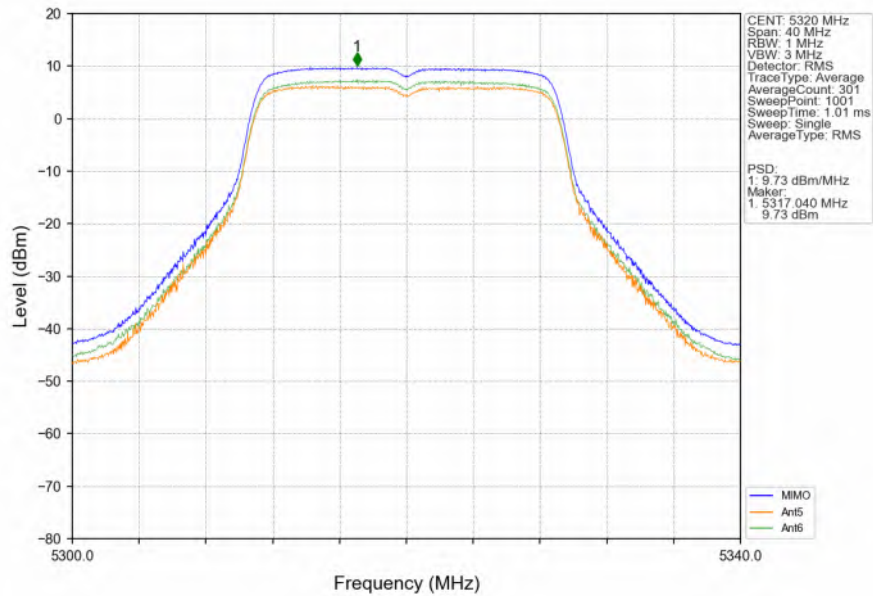
802.11n(HT20)_HCH_5320MHz_MIMO_NTNV
