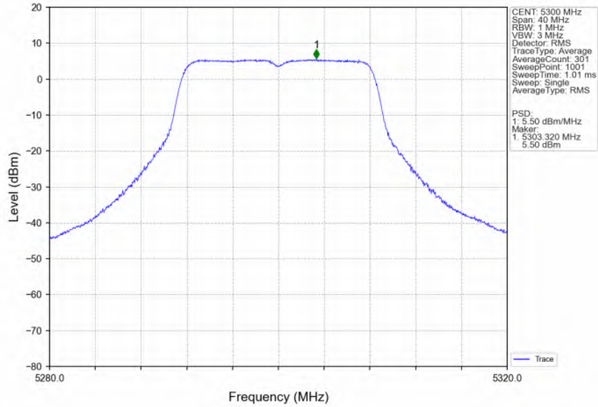
802.11a_MCH_5300MHz_Ant6_NTNV
