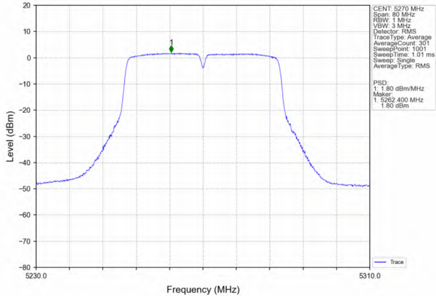
802.11n(HT40)_LCH_5270MHz_Ant6_NTNV
