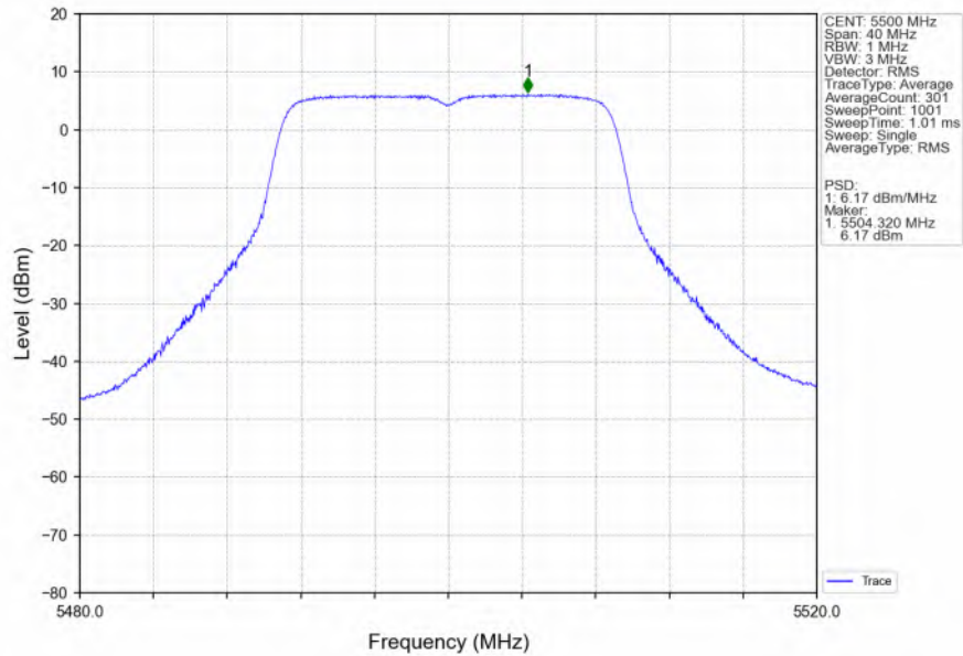
802.11n(HT20)_LCH_5500MHz_Ant6_NTNV
