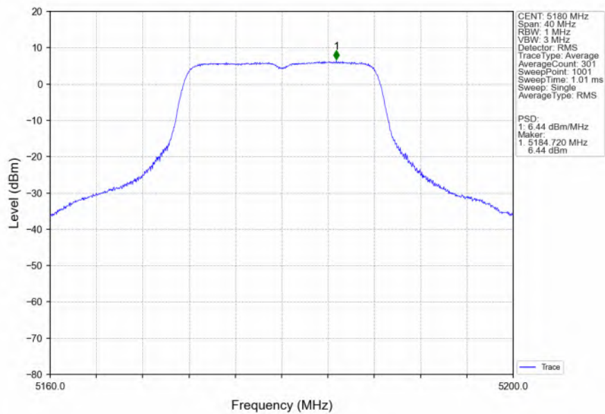
802.11a_LCH_5180MHz_Ant6_NTNV
