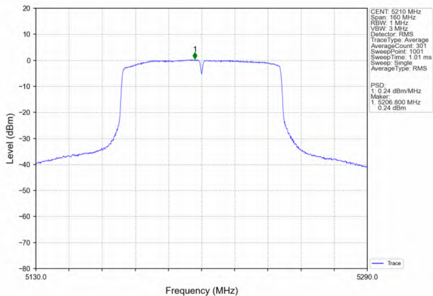
802.11ac(VHT80)_MCH_5210MHz_Ant6_NTNV
