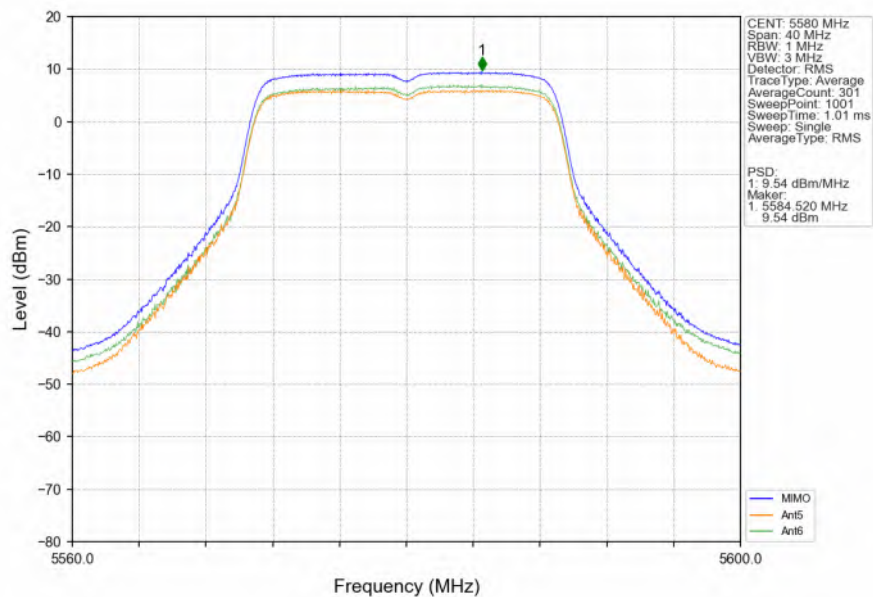
802.11n(HT20)_MCH_5580MHz_MIMO_NTNV
