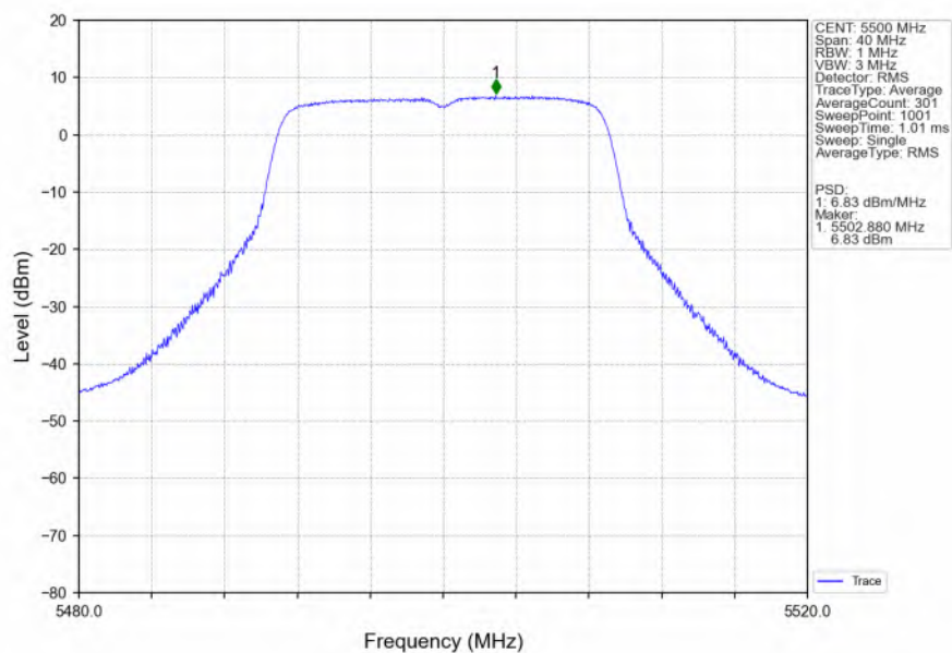
802.11ac(VHT20)_LCH_5500MHz_Ant6_NTNV
