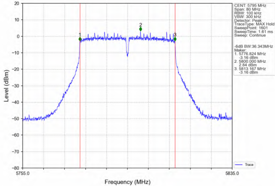
802.11n(HT40)_HCH_5795MHz_Ant6_NTNV
