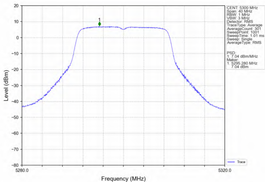
802.11n(HT20)_MCH_5300MHz_Ant6_NTNV
