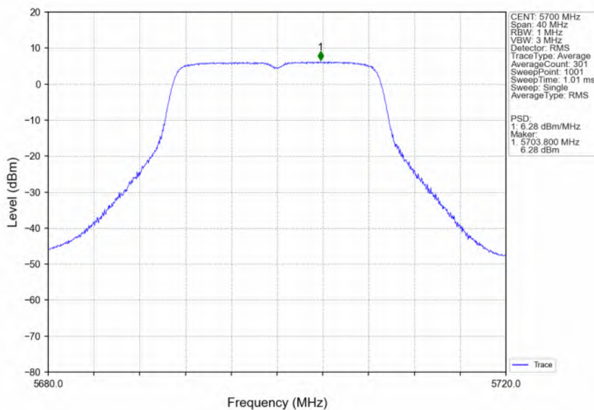
802.11n(HT20)_HCH_5700MHz_Ant6_NTNV
