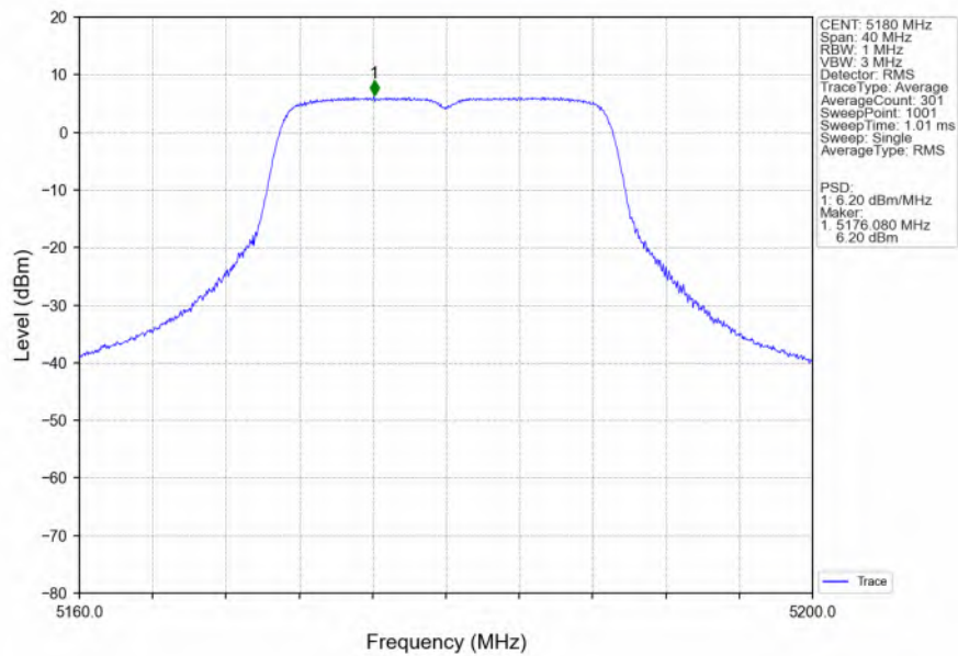
802.11n(HT20)_LCH_5180MHz_Ant6_NTNV
