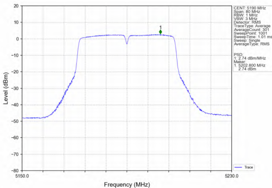
802.11n(HT40)_LCH_5190MHz_Ant6_NTNV
