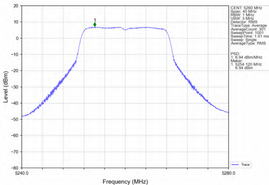
802.11a_LCH_5260MHz_Ant6_NTNV
