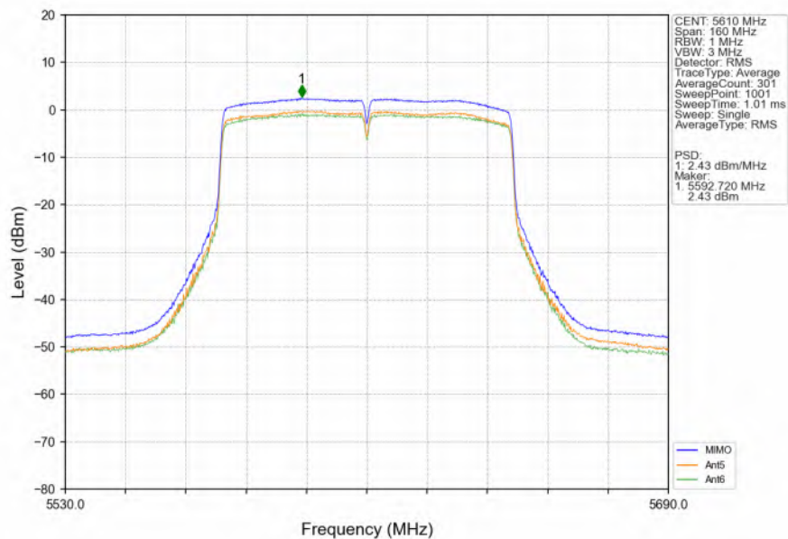
802.11ac(VHT80)_HCH_5610MHz_MIMO_NTNV
