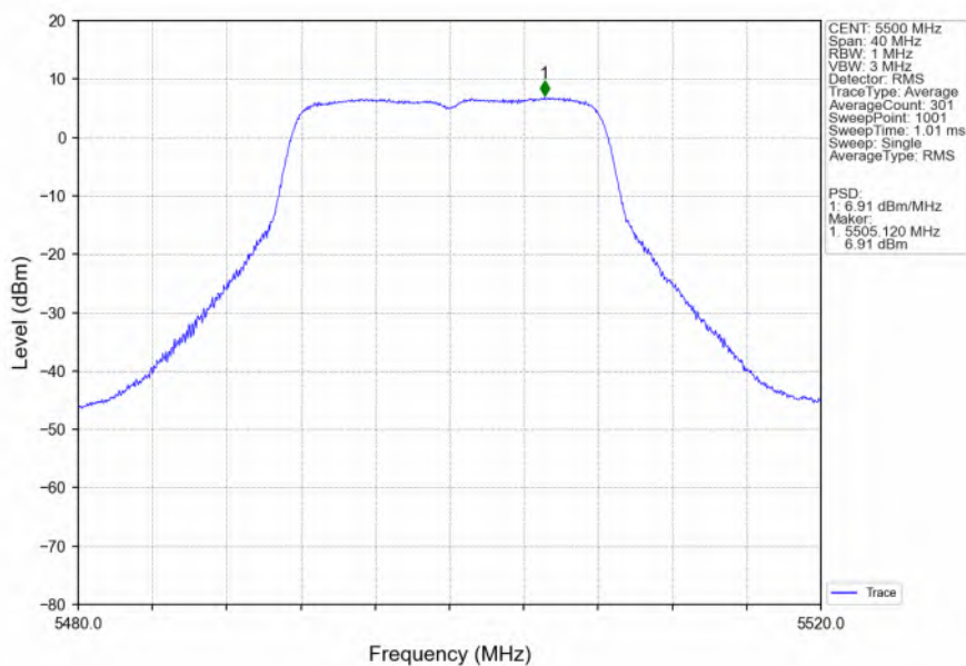
802.11a_LCH_5500MHz_Ant6_NTNV
