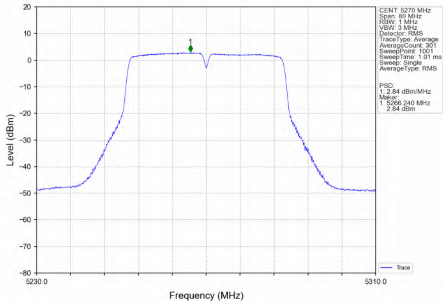
802.11n(HT40)_LCH_5270MHz_Ant6_NTNV
