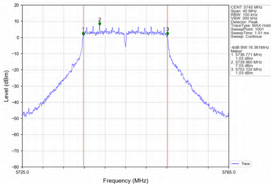
802.11a_LCH_5745MHz_Ant6_NTNV
