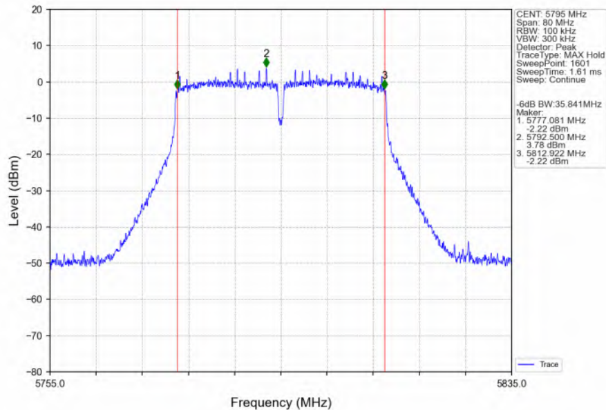
802.11n(HT40)_HCH_5795MHz_Ant6_NTNV
