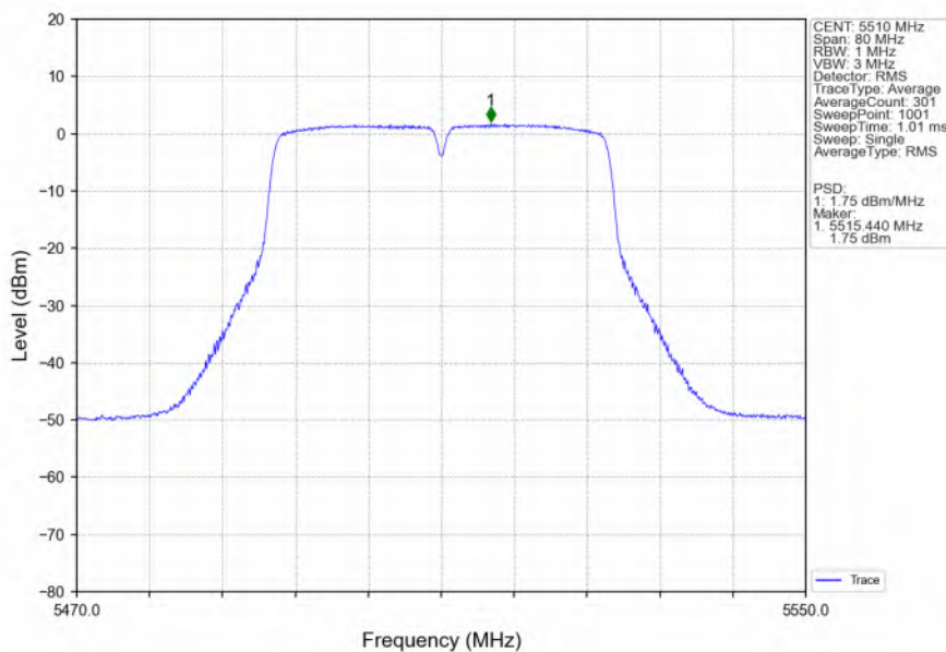
802.11n(HT40)_LCH_5510MHz_Ant6_NTNV
