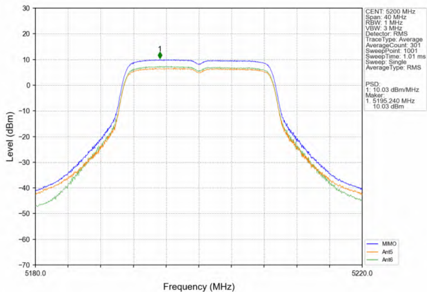
802.11n(HT20)_MCH_5200MHz_MIMO_NTNV
