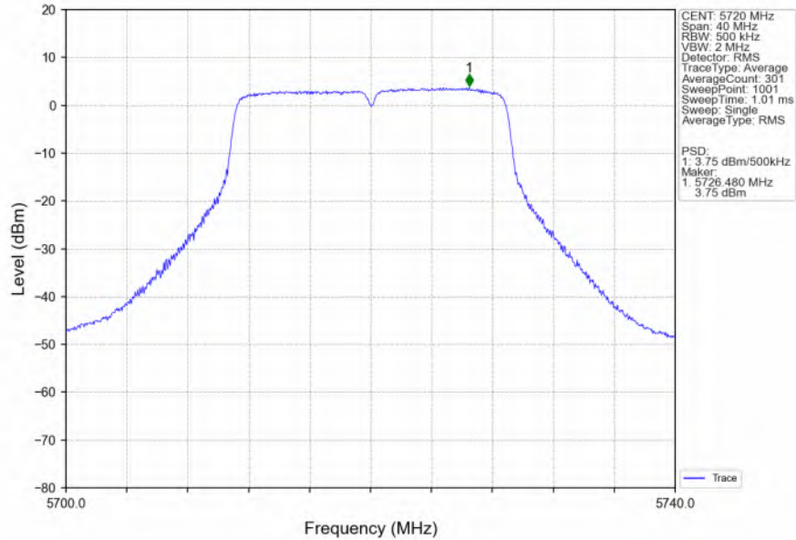
802.11n(HT20)_HCH_5720MHz_MIMO_NTNV
