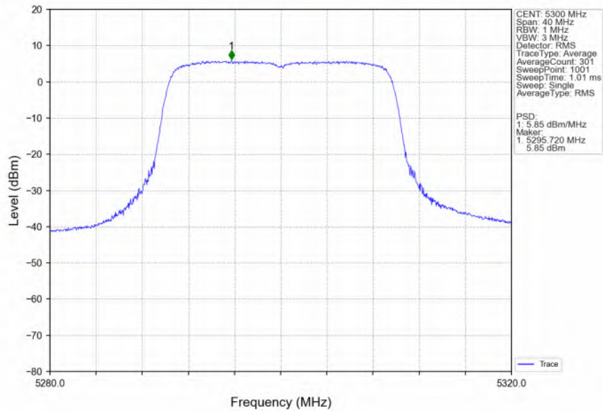
802.11be(EHT20)_MCH_5300MHz_SU_/_Ant6_NTNV
