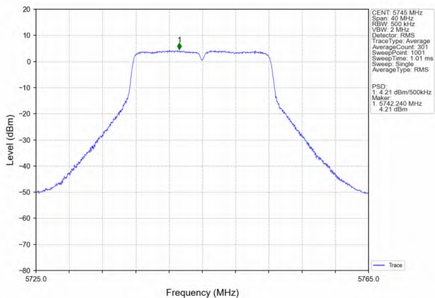
802.11a_LCH_5745MHz_Ant6_NTNV
