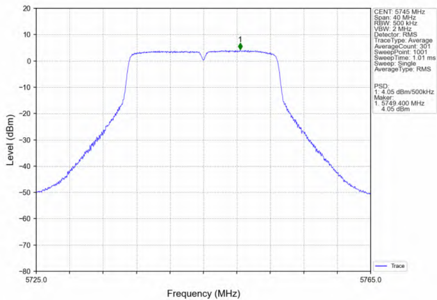
802.11n(HT20)_LCH_5745MHz_Ant6_NTNV
