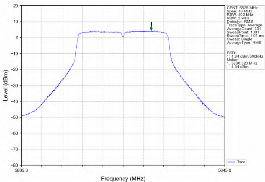
802.11n(HT20)_HCH_5825MHz_Ant6_NTNV
