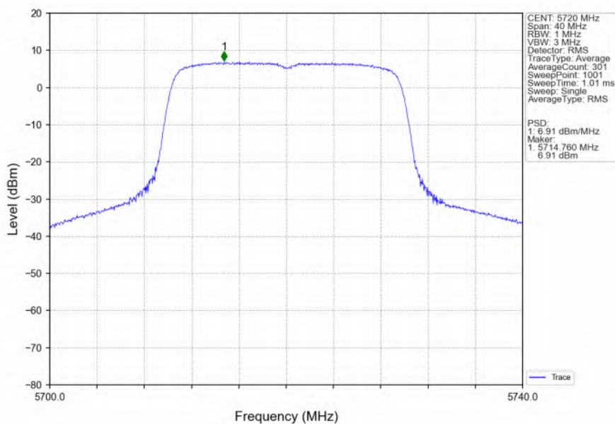
802.11ax(HEW20)_HCH_5720MHz_SU_ / _Ant6_NTNV
