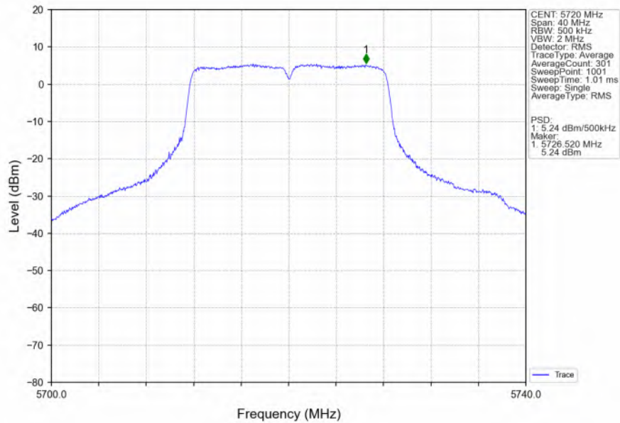
802.11a_HCH_5720MHz_Ant6_NTNV
