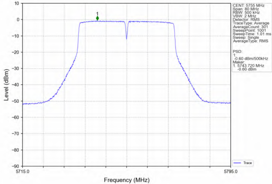
802.11ac(VHT40)_LCH_5755MHz_MIMO_NTNV
