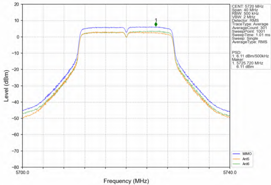
802.11n(HT20)_HCH_5720MHz_MIMO_NTNV
