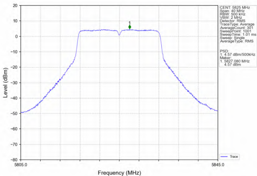
802.11a_HCH_5825MHz_Ant6_NTNV
