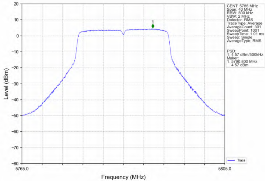
802.11n(HT20)_MCH_5785MHz_MIMO_NTNV
