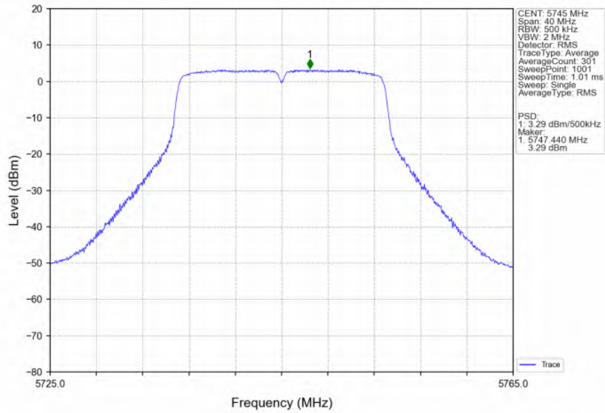
802.11n(HT20)_LCH_5745MHz_Ant6_NTNV
