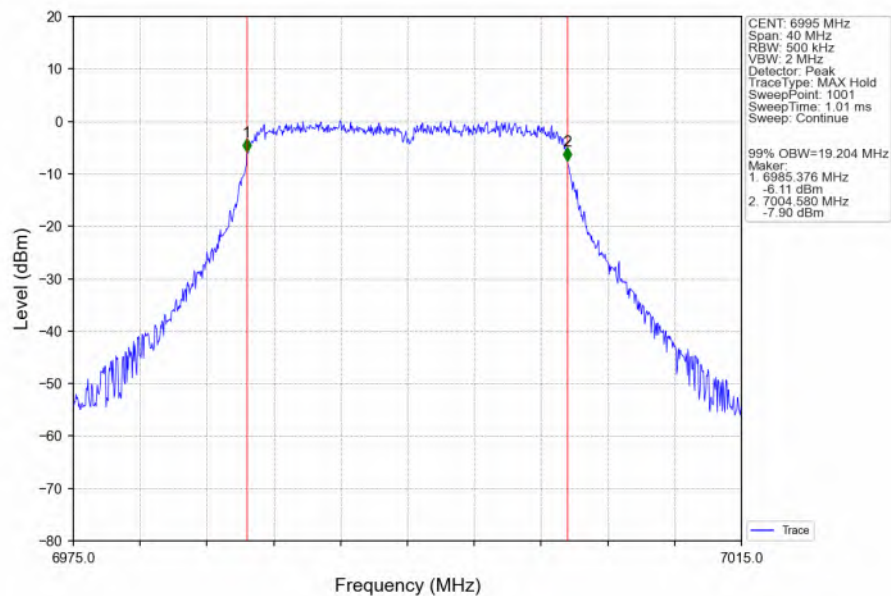
802.11be(EHT20)_MCH_6995MHz_SU_ / _Ant1_NTNV
