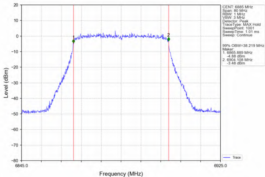
802.11be(EHT40)_HCH_6885MHz_SU_/_Ant1_NTNV
