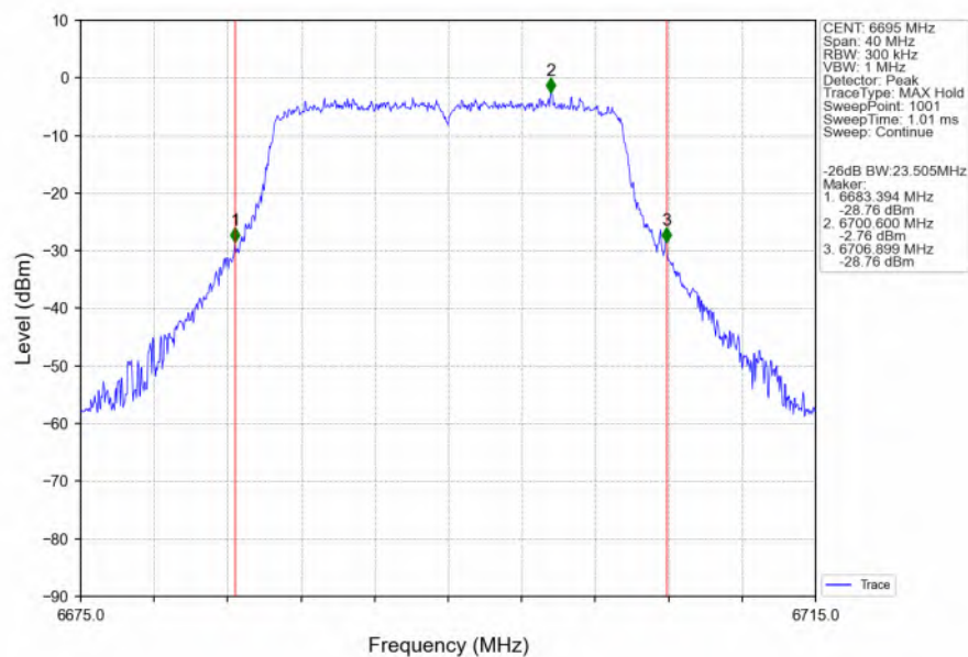
802.11be(EHT20)_MCH_6695MHz_SU_/_Ant1_NTNV
