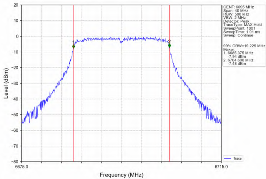
802.11be(EHT20)_MCH_6695MHz_SU_/_Ant1_NTNV
