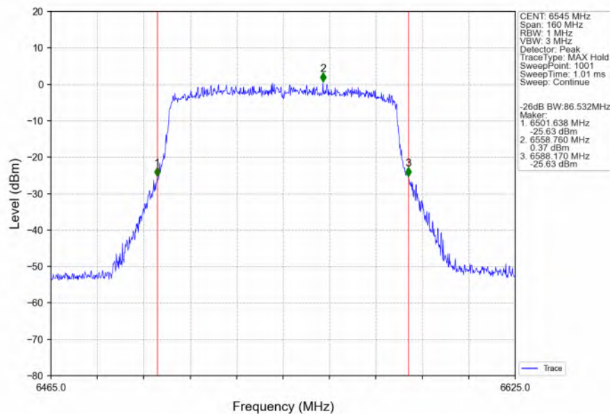
802.11be(EHT80)_HCH_6545MHz_SU_/_Ant1_NTNV
