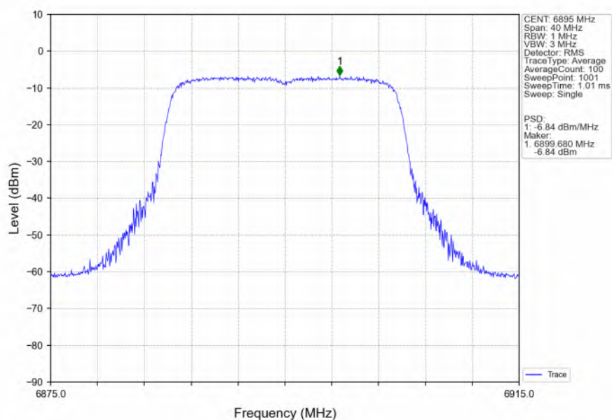
802.11be(EHT20)_LCH_6895MHz_SU_/_Ant2_NTNV
