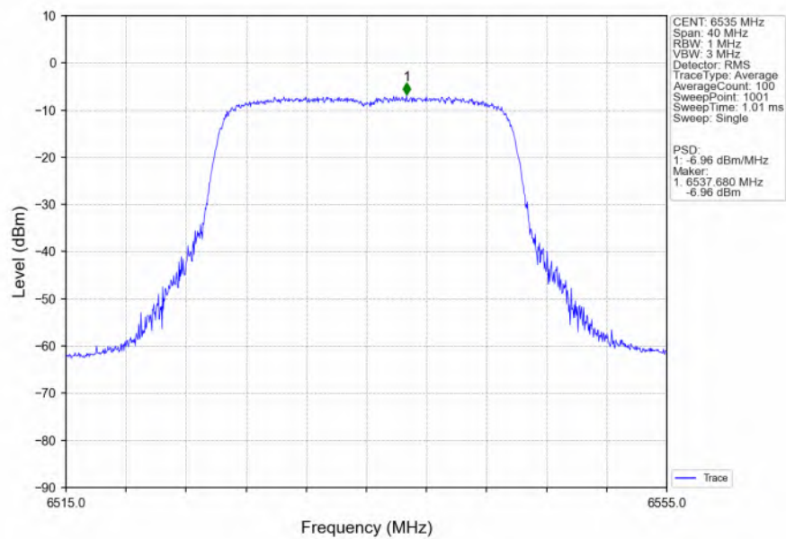
802.11be(EHT20)_LCH_6535MHz_SU_/_Ant2_NTNV
