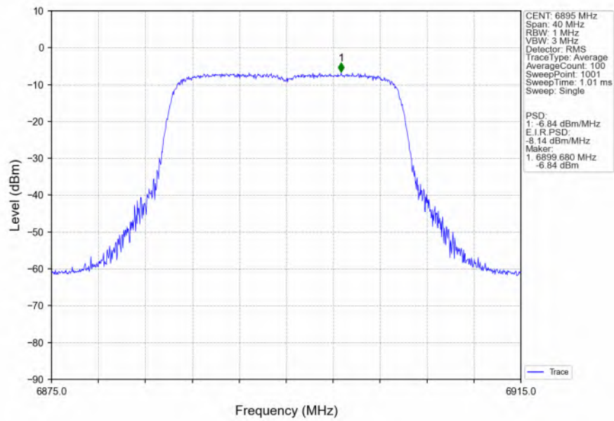
802.11be(EHT20)_LCH_6895MHz_SU_/_Ant2_NTNV
