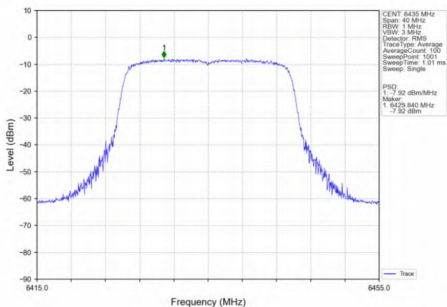
802.11be(EHT20)_LCH_6435MHz_SU_/_Ant2_NTNV
