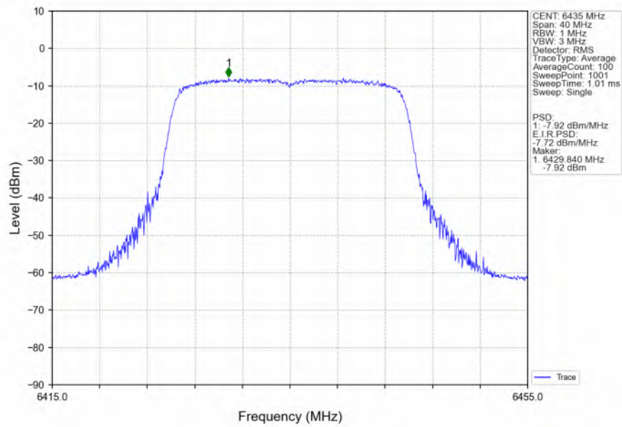
802.11be(EHT20)_LCH_6435MHz_SU_/_Ant2_NTNV
