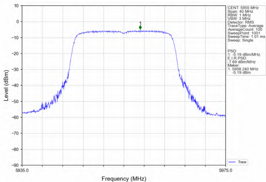
802.11be(EHT20)_LCH_5955MHz_SU_/_Ant2_NTNV
