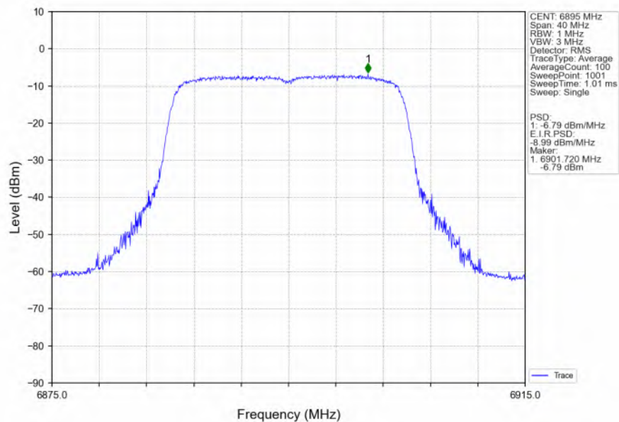
802.11be(EHT20)_LCH_6895MHz_SU_/_Ant2_NTNV
