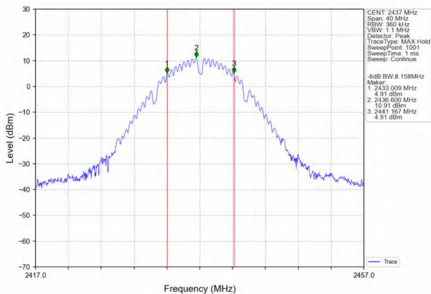
802.11b_MCH_2437MHz_Ant5 (SISO)_NTNV
