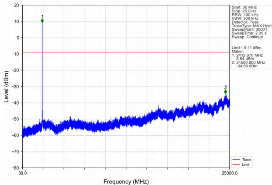
802.11b_LCH_2412MHz_Ant5 (SISO)_NTNV
