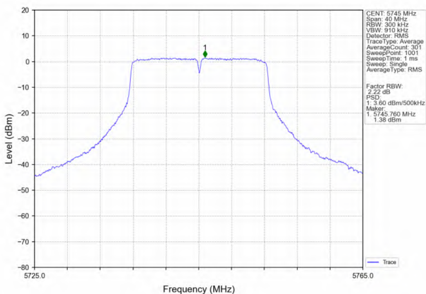
802.11a_LCH_5745MHz_Ant6_NTNV
