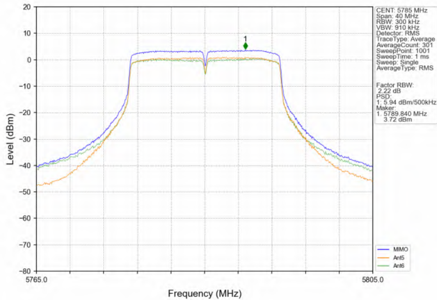
802.11n(HT20)_MCH_5785MHz_MIMO_NTNV
