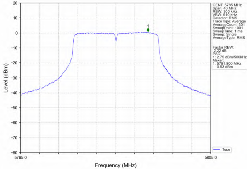
802.11n(HT20)_MCH_5785MHz_MIMO_NTNV
