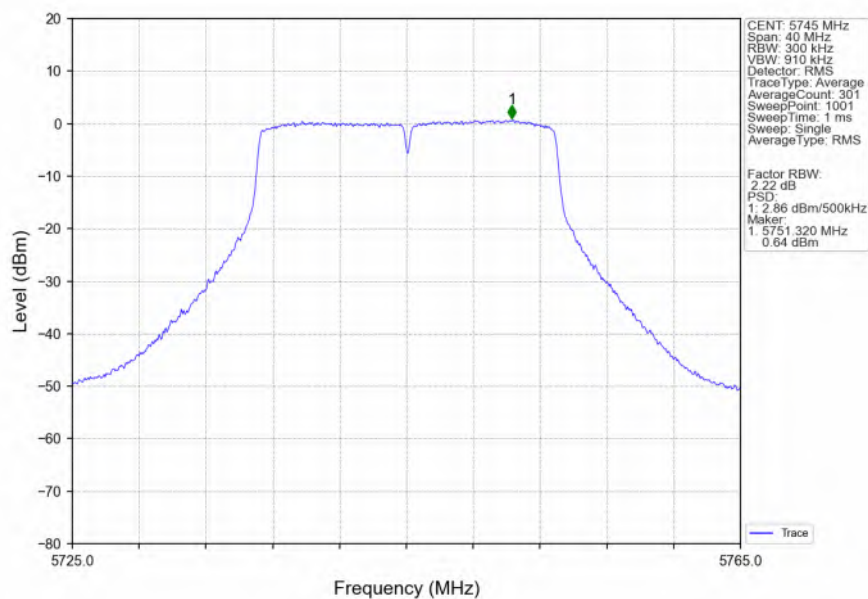
802.11n(HT20)_LCH_5745MHz_Ant6_NTNV
