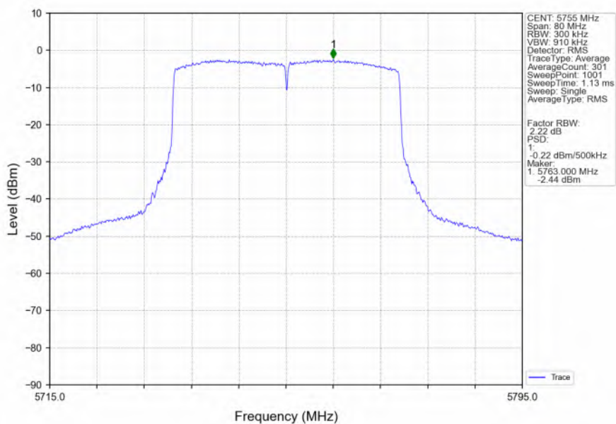
802.11be(EHT40)_LCH_5755MHz_SU_/_Ant6_NTNV
