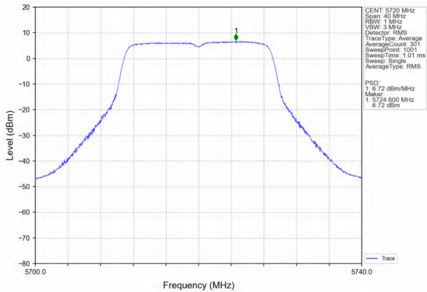
802.11ac(VHT20)_HCH_5720MHz_Ant6_NTNV
