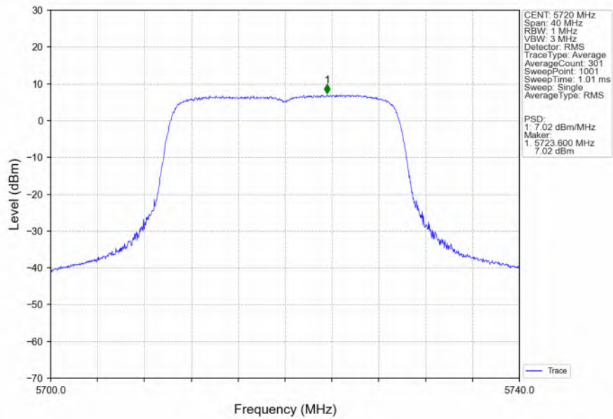
802.11be(EHT20)_HCH_5720MHz_SU_ / _Ant6_NTNV
