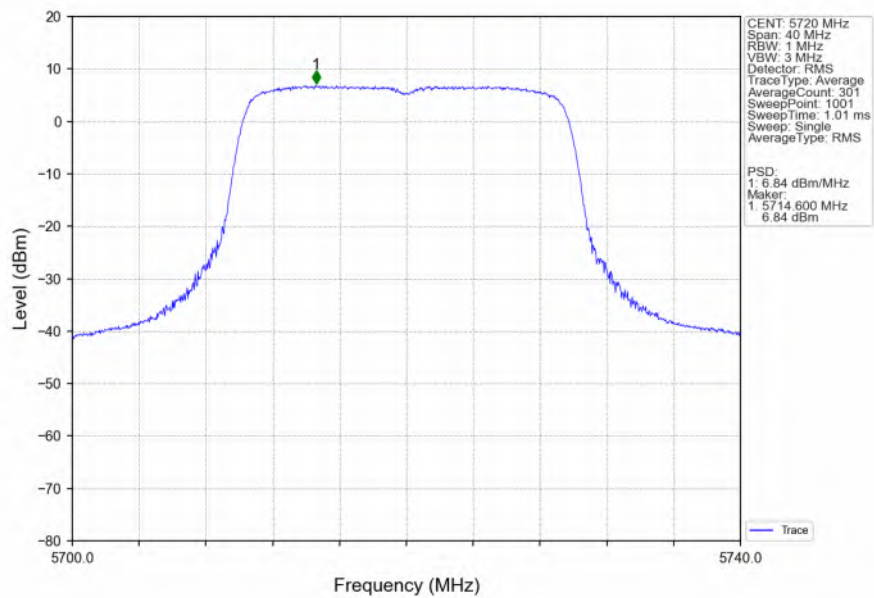
802.11be(EHT20)_HCH_5720MHz_SU_ / _MIMO_NTNV
