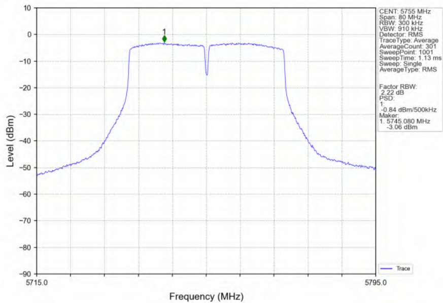
802.11n(HT40)_LCH_5755MHz_MIMO_NTNV
