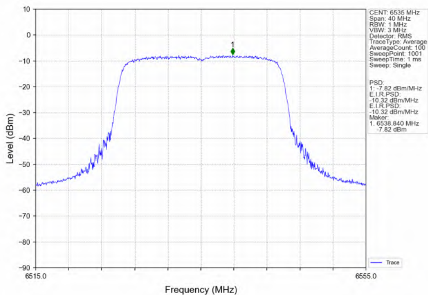
802.11be(EHT20)_LCH_6535MHz_SU / _Ant2_NTNV
