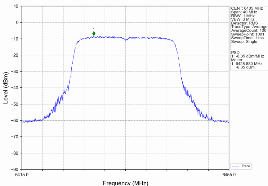
802.11be(EHT20)_LCH_6435MHz_SU / _Ant2_NTNV
