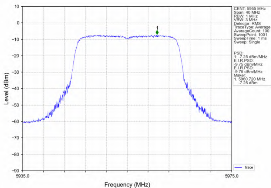
802.11be(EHT20)_LCH_5955MHz_SU / _Ant2_NTNV
