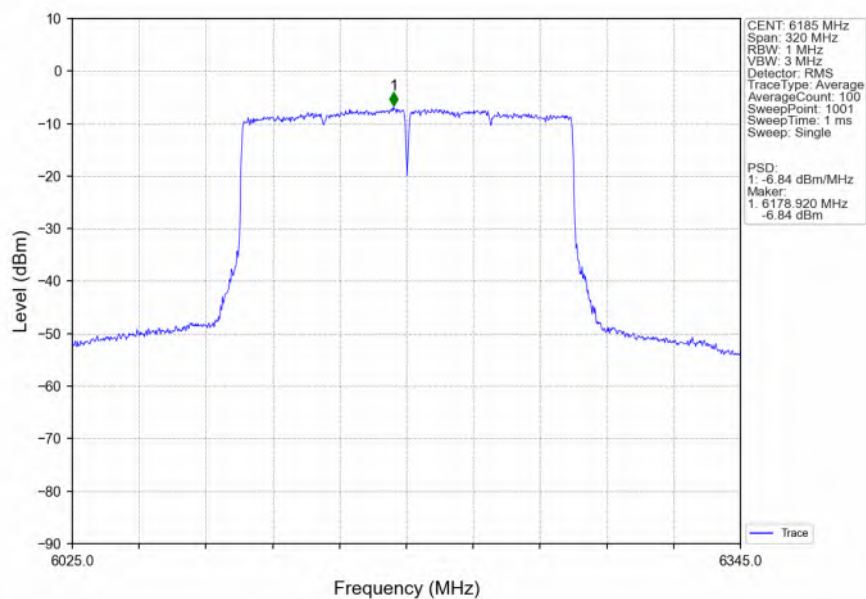
802.11be(EHT160) MCH 6185MHz SU / Ant2 NTN
