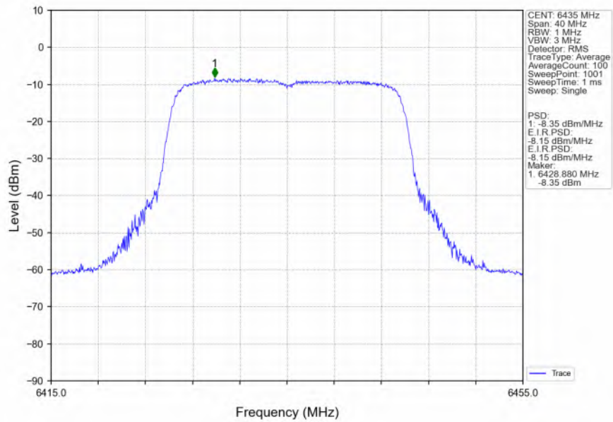
802.11be(EHT20)_LCH_6435MHz_SU / _Ant2_NTNV
