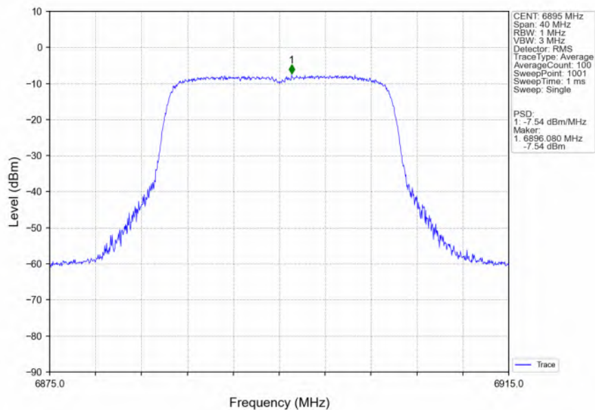
802.11be(EHT20)_LCH_6895MHz_SU / _Ant2_NTNV
