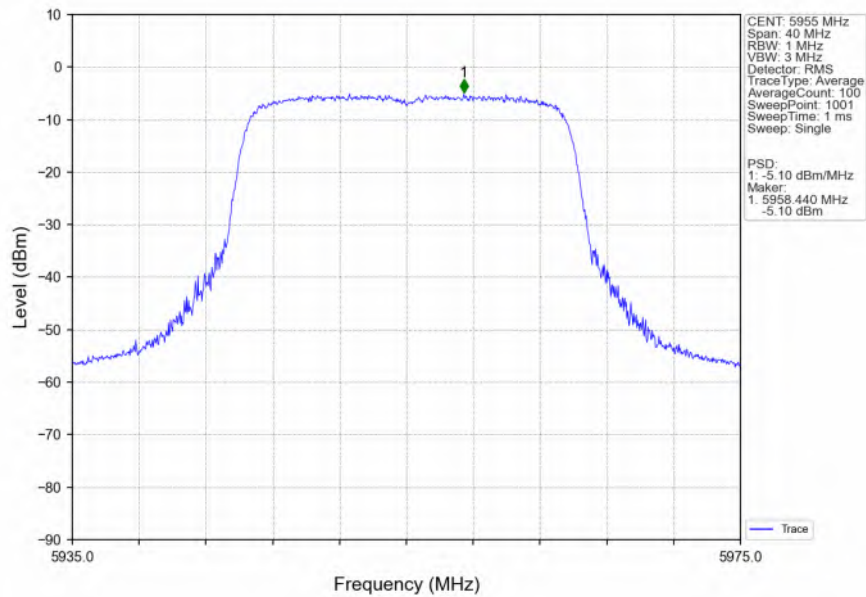
802.11be(EHT20)_LCH_5955MHz_SU_/_Ant2_NTNV
