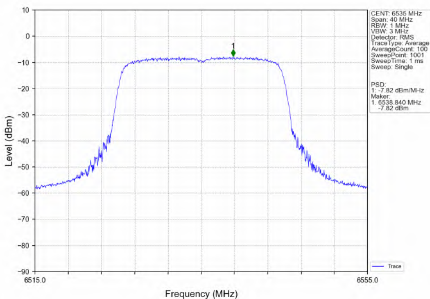
802.11be(EHT20)_LCH_6535MHz_SU / _Ant2_NTNV
