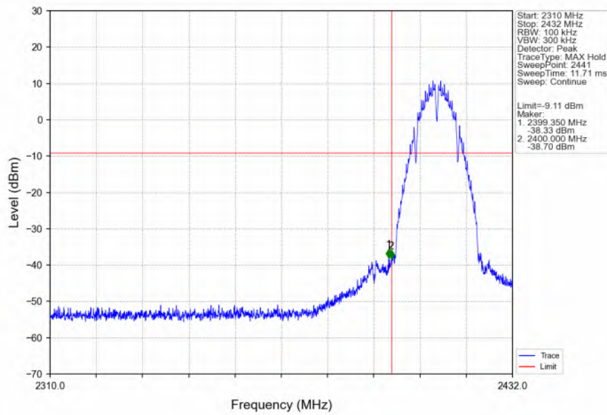
802.11b_LCH_2412MHz_Ant5 (SISO)_NTNV
