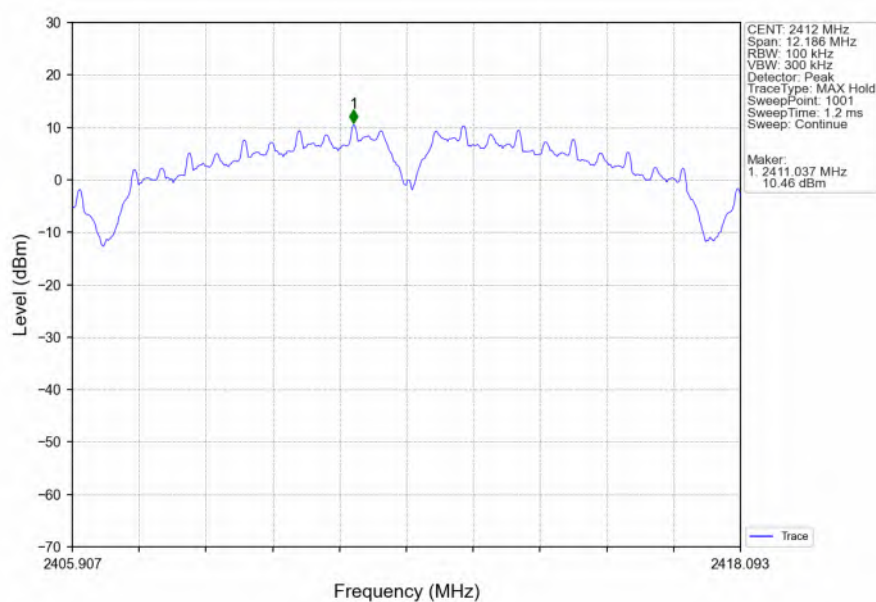
802.11b_LCH_2412MHz_Ant6 (SISO)_NTNV
