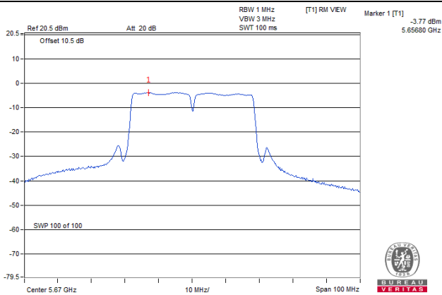
802.11n (40MHz)_Chain 0 / CH134
