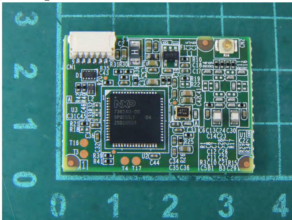
(31) EUT Photo_NFC Module
