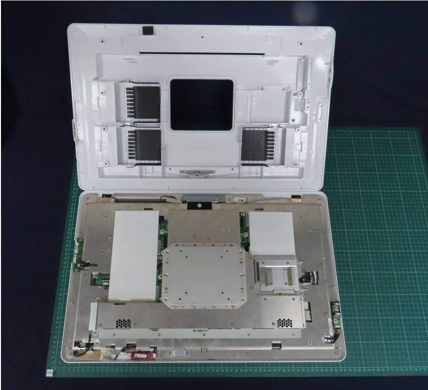
(5) EUT Photo
